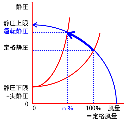
図 2.1.6.5-4 段数制御
