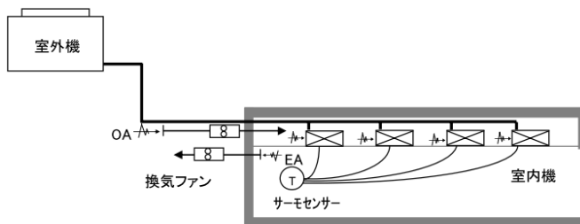
図 2.4.1.2-1 計算モデル
