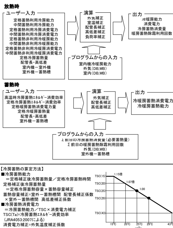
図 2.4.4-4 氷蓄熱ビル用マルチエアコンの計算モデルの概
