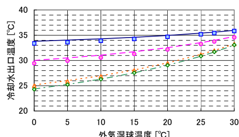
図 2.4.3-6 変風量時の冷却水出口温度 (圧縮用、開放型、冷却水入口温度 37°C)
