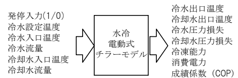
図 2.4.2.1-10 水冷式ヒートポンプチラーの入出力
