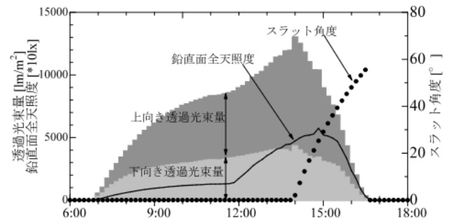
図 2.2.1.5-3 ブラインド自動制御下における窓透過光束量の指向性
