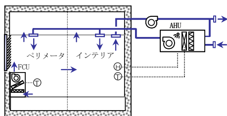
図 2.2.1.1-4 空調システム
