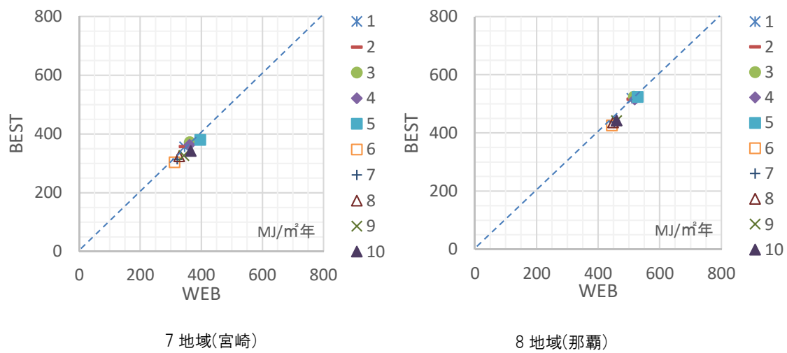
図 4.4.1.5)-2 学校 各ケースの PAL*[MJ/m²年]
