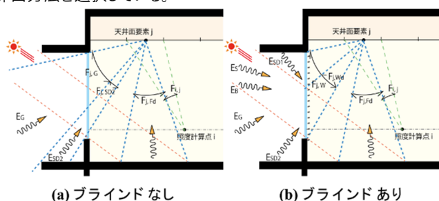
図 2.2.1.5-1 間接照度計算模式図
