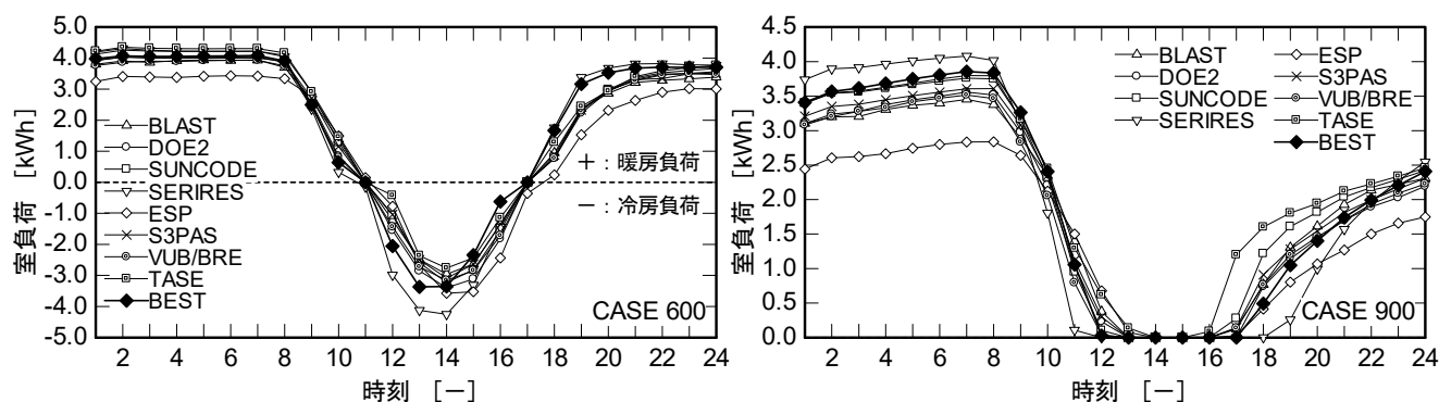
図 1.2.3.2-8 1月4日の室負荷の時刻変動による比較(左:CASE_600、右:CASE_900)
