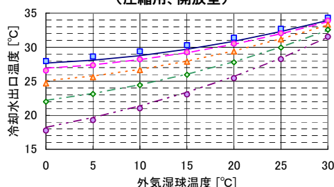
図 2.4.3-4 定格時の冷却水出口温度 (圧縮用、開放型)
