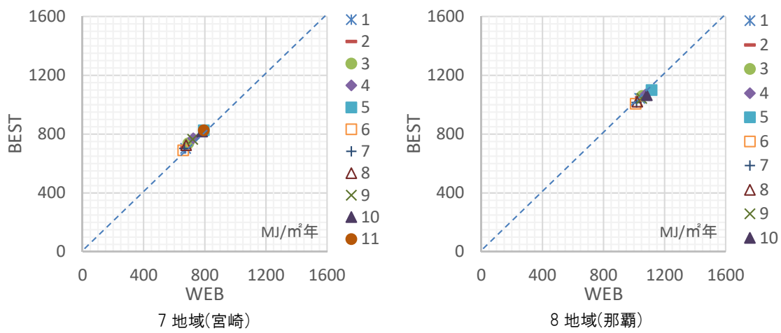
図 4.4.1.8)-2 体育館 各ケースの PAL* [MJ/m²年]
