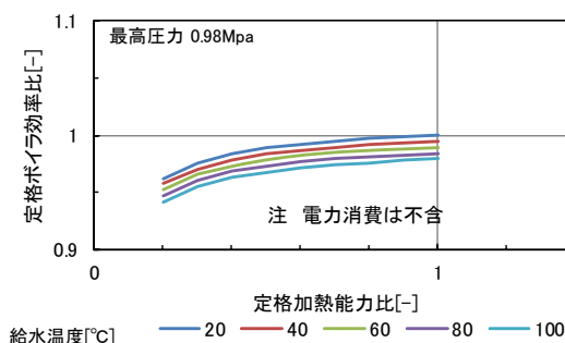
図 2.4.2.3-2 真空温水器の機器特
