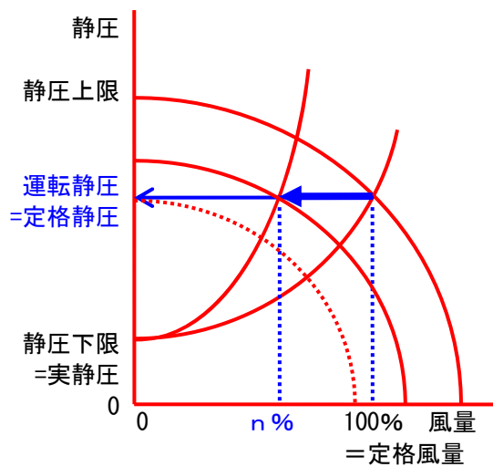
図 2.1.6.5-5 吐出圧一定制御
