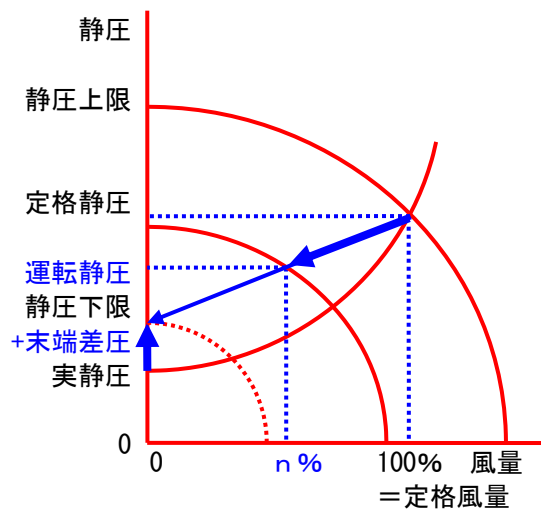
図 2.1.6.5-7 推定末端差圧制御
