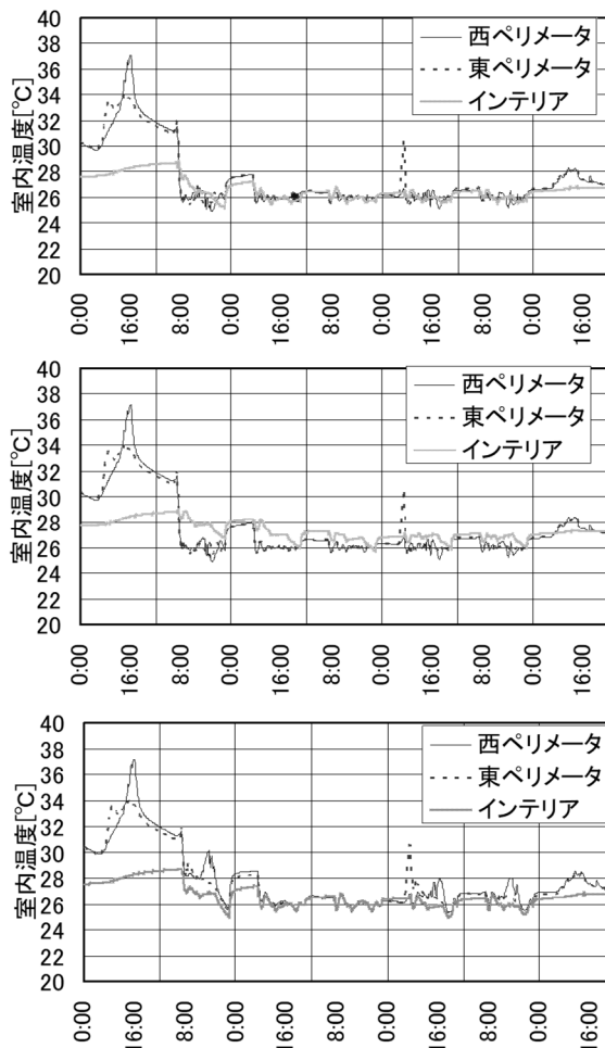
図 2.2.1.3-5 計算結果
