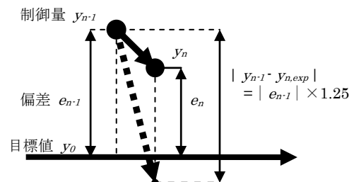
図 2.3.1.4-2 比例ゲインの調整法
