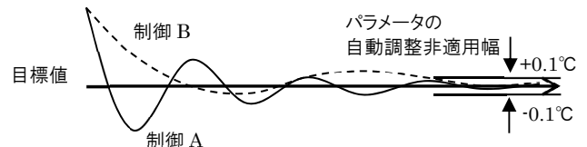
図 2.3.1.4-1 比例ゲインの自動調整時の制御
