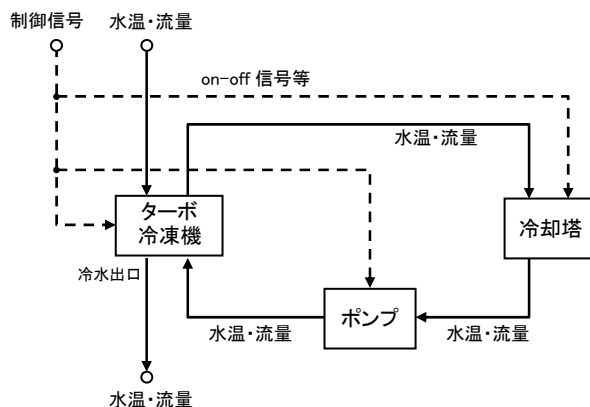
図 2.3.1.3-6 熱源システムにおけるモジュール接続と水温・水量の流れ
