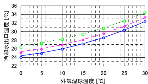
図 2.4.3-4 定格時の冷却水出口温度 (圧縮用、開放型)
