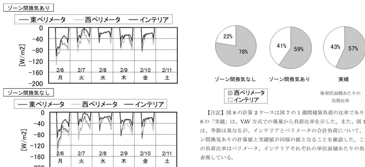
図 2.2.1.3-4 インテリア・ペリメータ負荷比率
