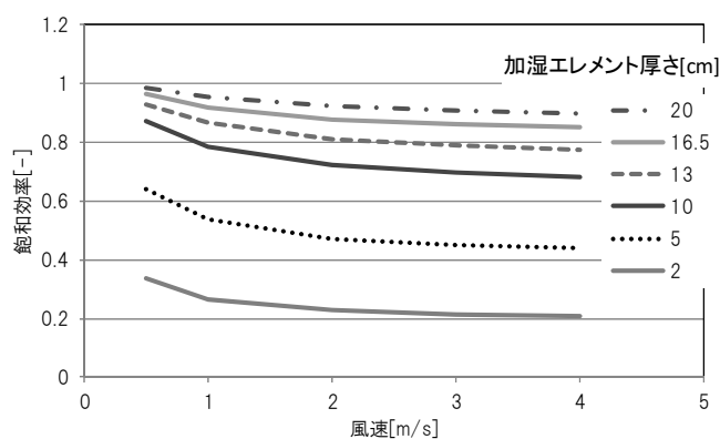
図 2.4.6-6 気化式加湿器機器特性
