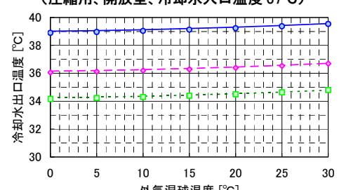
図 2.4.3-6 変風量時の冷却水出口温度 (圧縮用、開放型、冷却水入口温度 37°C)
