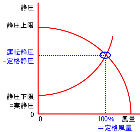
図 2.1.6.5-3 定流量
