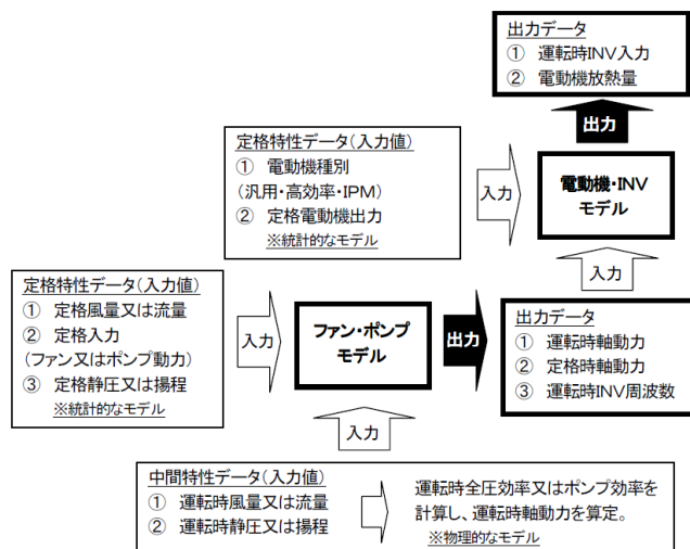
図 2.4.1.1-6 搬送機器(ファン・ポンプ)のモデル化の概要
