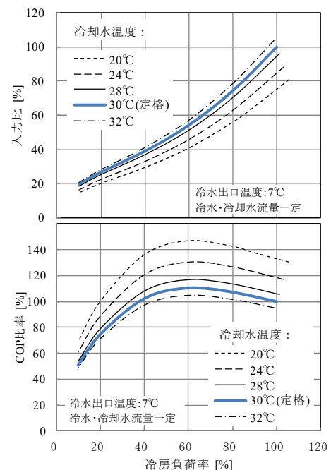
図 2.4.2.1-12 水冷チラー/スクリーの部分負荷特性
