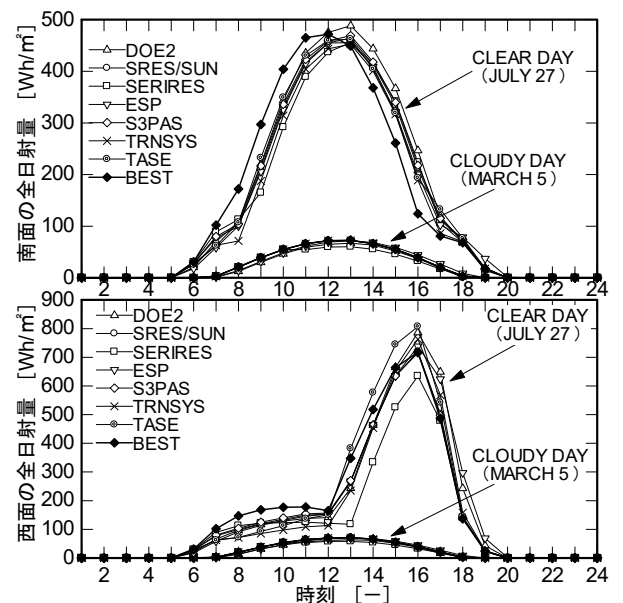
図 1.2.3.2-6 全日射量の時刻変動による比較
