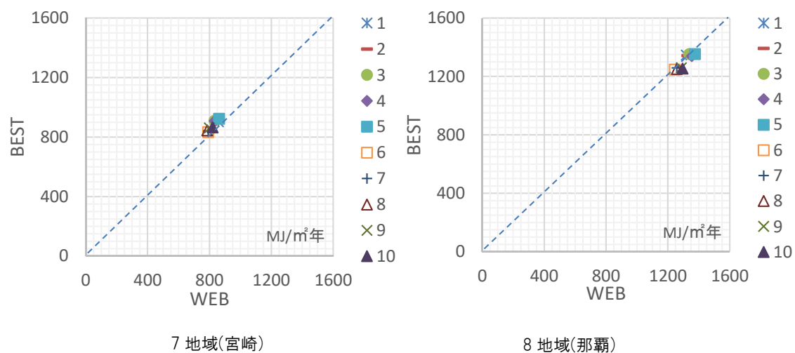
図 4.4.1.4)-2 物販店舗 各ケースの PAL*[MJ/m²年]
