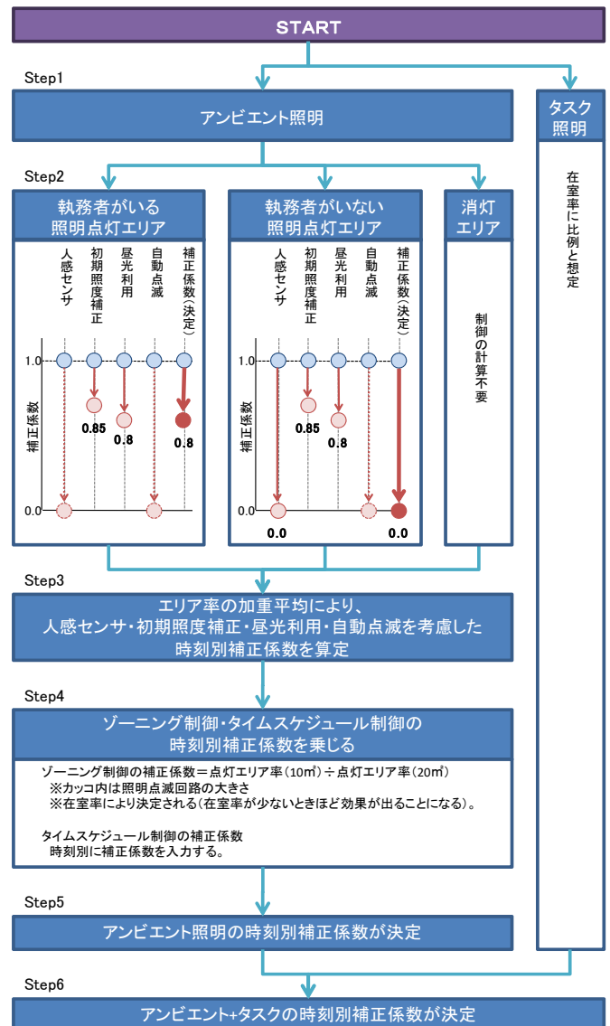
図 2.2.1.6-4 複数の照明制御を導入した場合の照明発熱の計算方法
