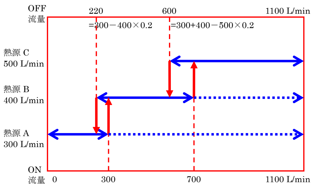
図 5-36 台数制御の例 [流量による制御 定格流量 A=300、B=400、C=500L/min]
