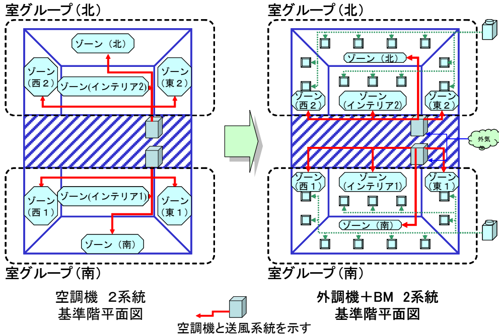
図 3-87 空調系統の変更内容
