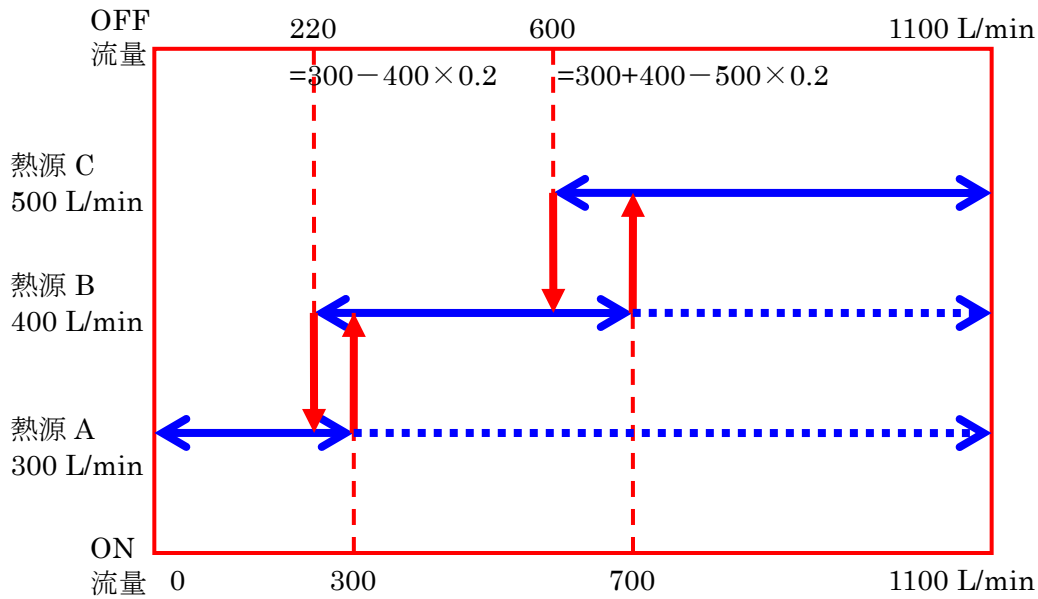
図 5-42 台数制御の例 [流量による制御 定格流量 A=300、B=400、C=500L/min]
