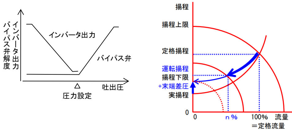
図 4-37. 推定末端差圧一定制御の概要
