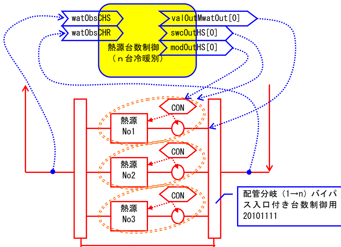
図 5-40 ノードの接続例 熱源群
