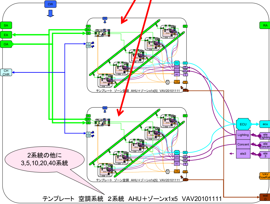
図 4-24 テンプレート 空調システム 2系統 AHU+ゾーン x1x5 VAV20101111
