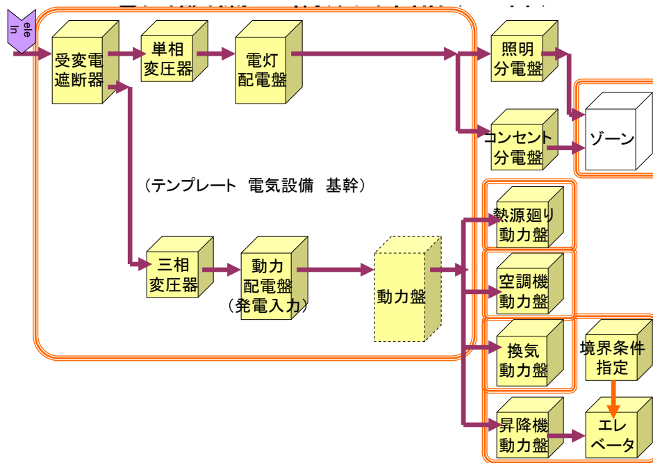
図 3-62 電気設備の構成部品(基幹)
