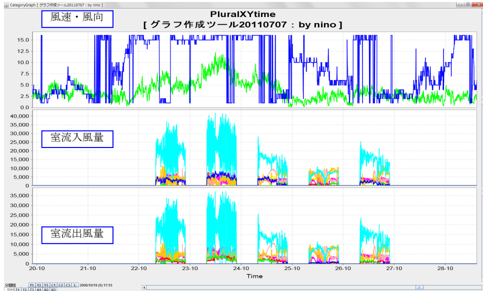
図 5-15 計算結果(2)
