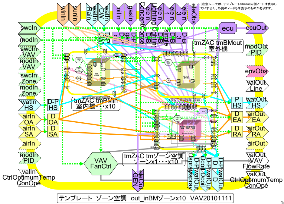
図 4-21「ゾーン空調テンプレート」の内部構成の参考詳細図(3)
