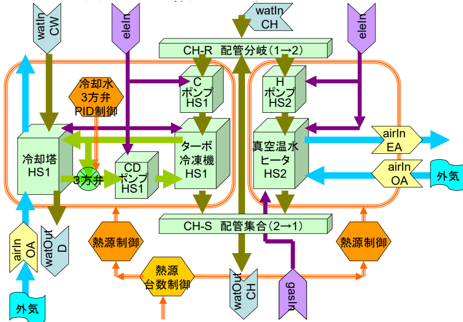
図 3-79 熱源廻りの構成部品(モジュール)
