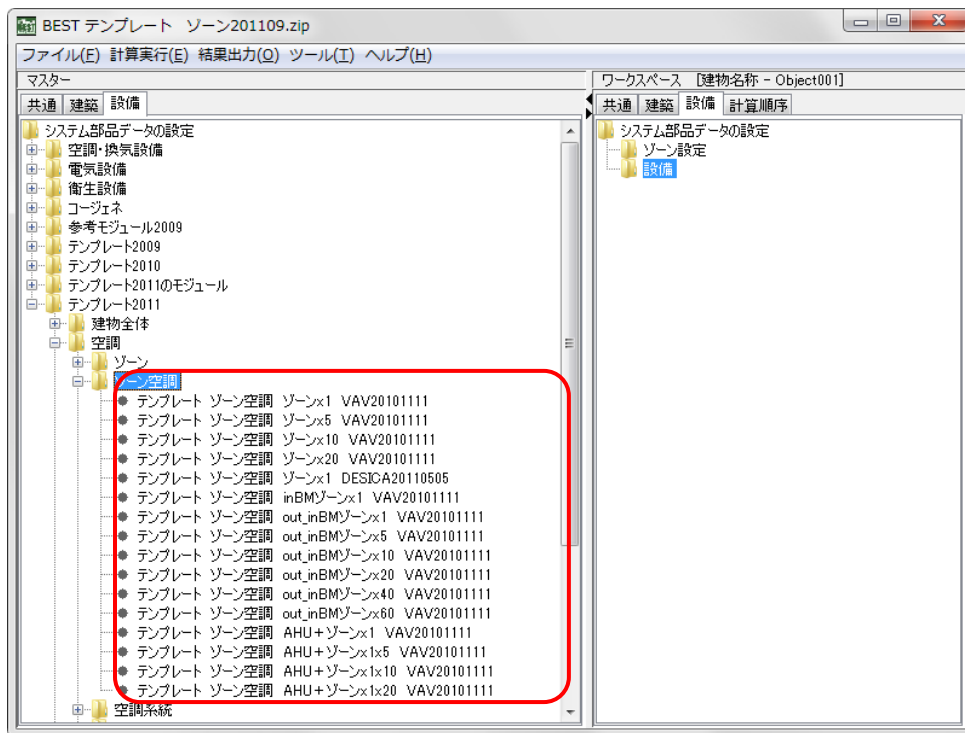
図 4-11「ゾーン空調」テンプレートの実装例（プログラム実行画面より）
