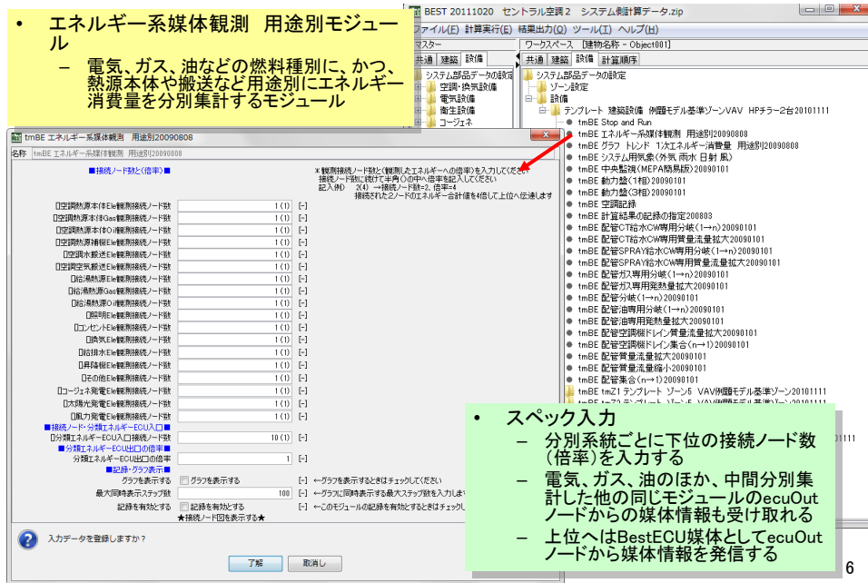
図 3-11 建物全体テンプレート直下の主なモジュール(3)
