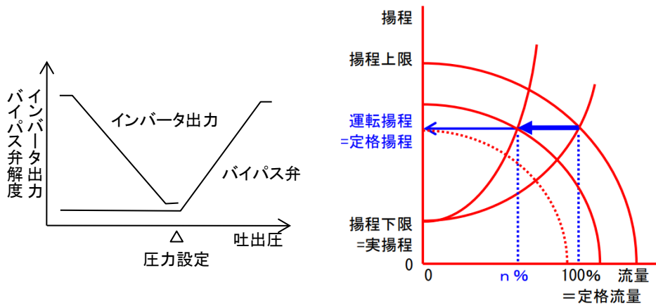
図 4-35. 吐出圧一定制御の概要
