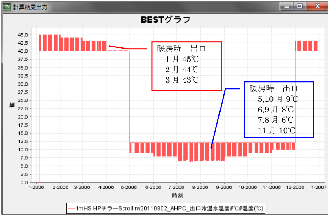
図 5-31 熱源 (HP チラー) の月別目標温度での計算結果 年間熱源出口冷温水温度
