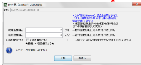
図 3-38 空調機テンプレート構成モジュール(11)
