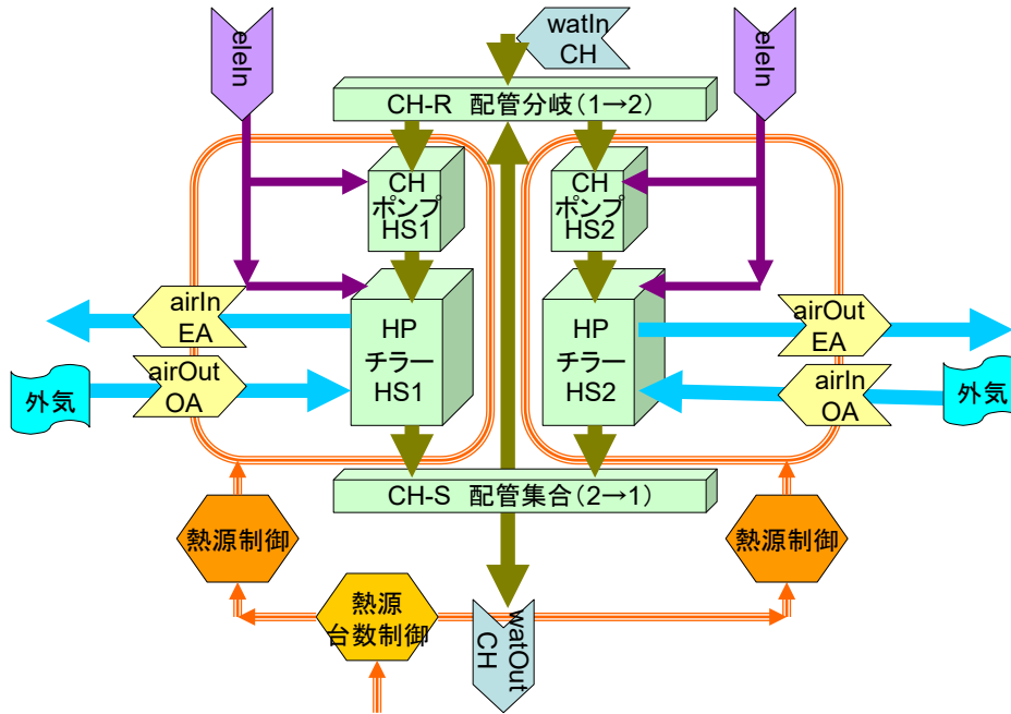
図 3-63 熱源廻りの構成部品 (モジュール)
