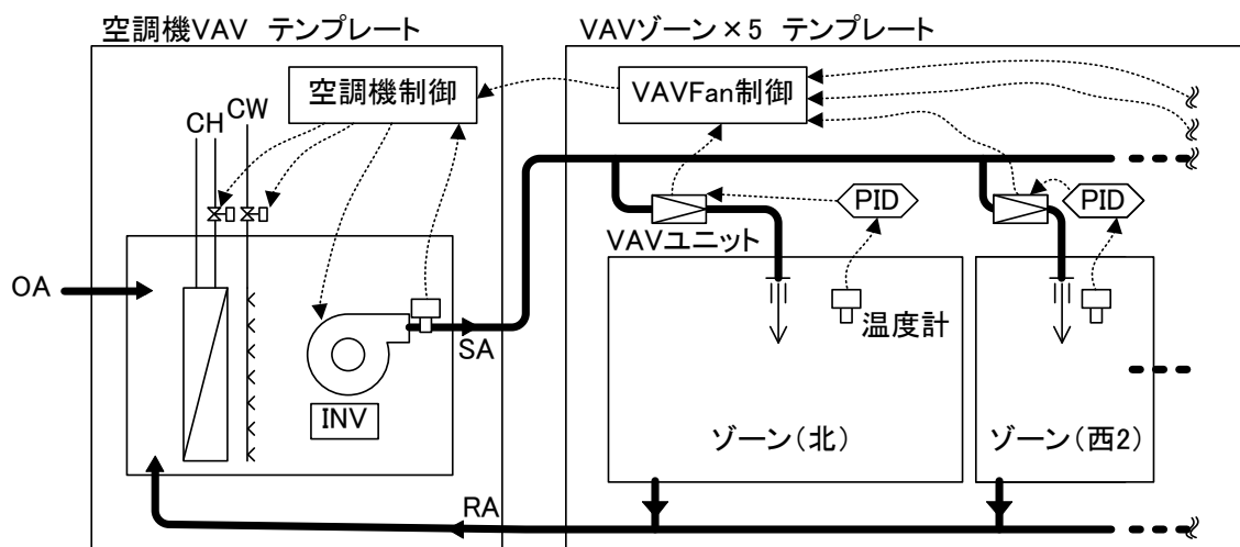
図 3-81 VAV システムのテンプレートにおける接続
