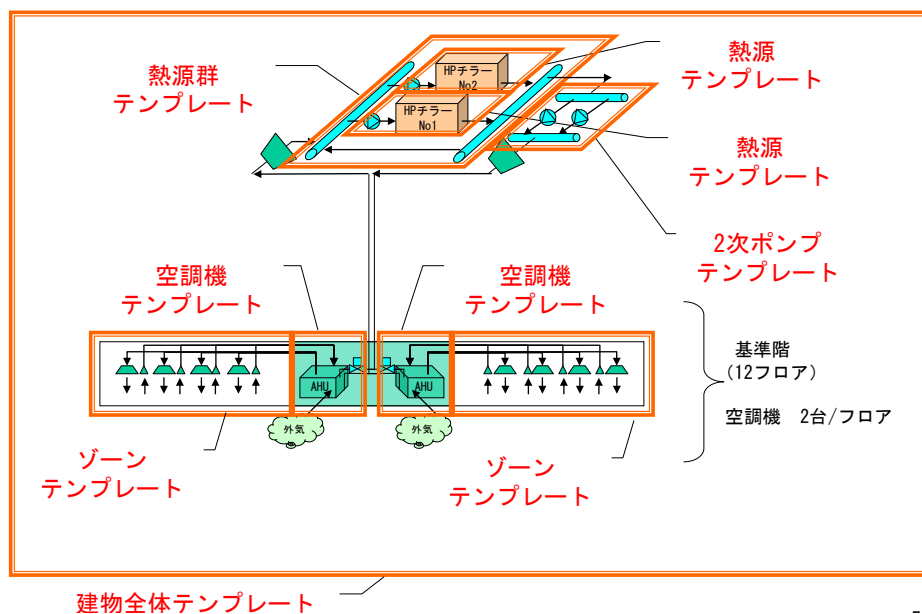
図 3-5 2次側空調設備と熱源(テンプレート)
