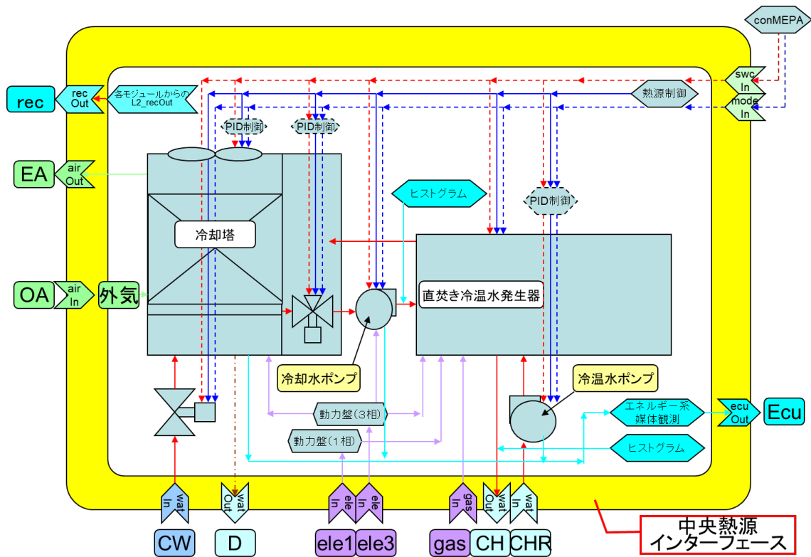
図 4-42「熱源テンプレート」の内部構成の参考詳細図（直焚き冷温水発生機）
