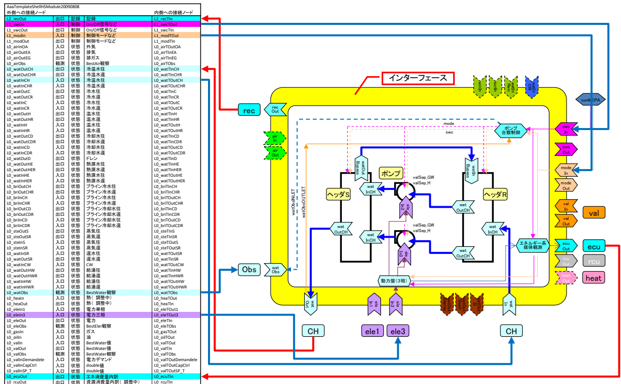
図 4-33. テンプレート「2次ポンプ」の Shell と内部モジュールとのノード接続情報
