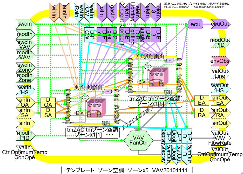
図 4-19「ゾーン空調テンプレート」の内部構成の参考詳細図(1)
