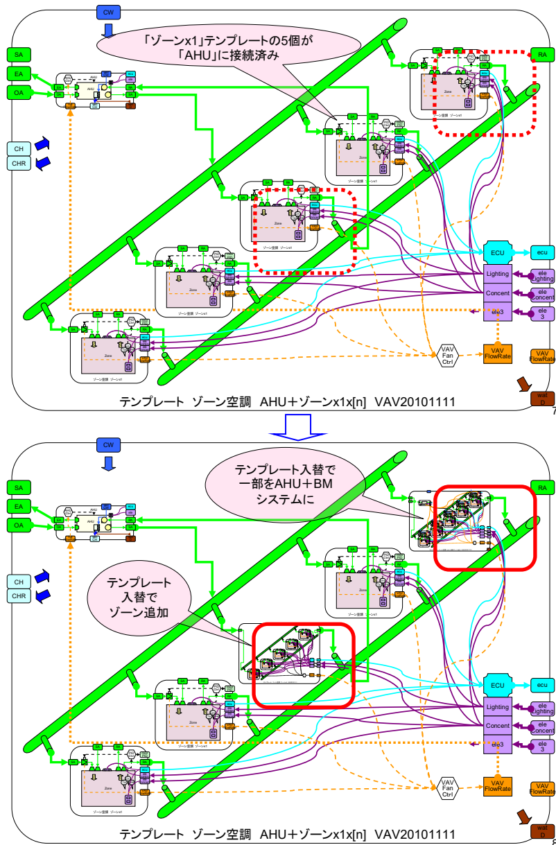
図 4-18 複雑なシステムへの展開例
