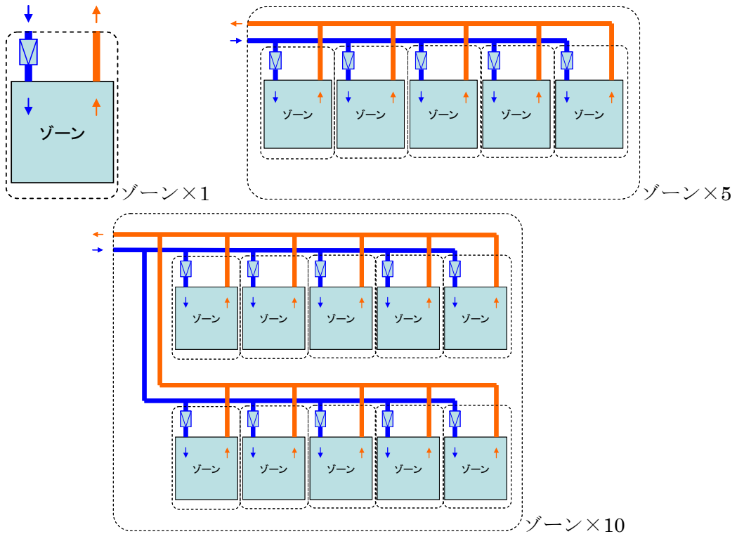
図 4-5 ゾーンのみで構成するゾーン空調テンプレートの例
