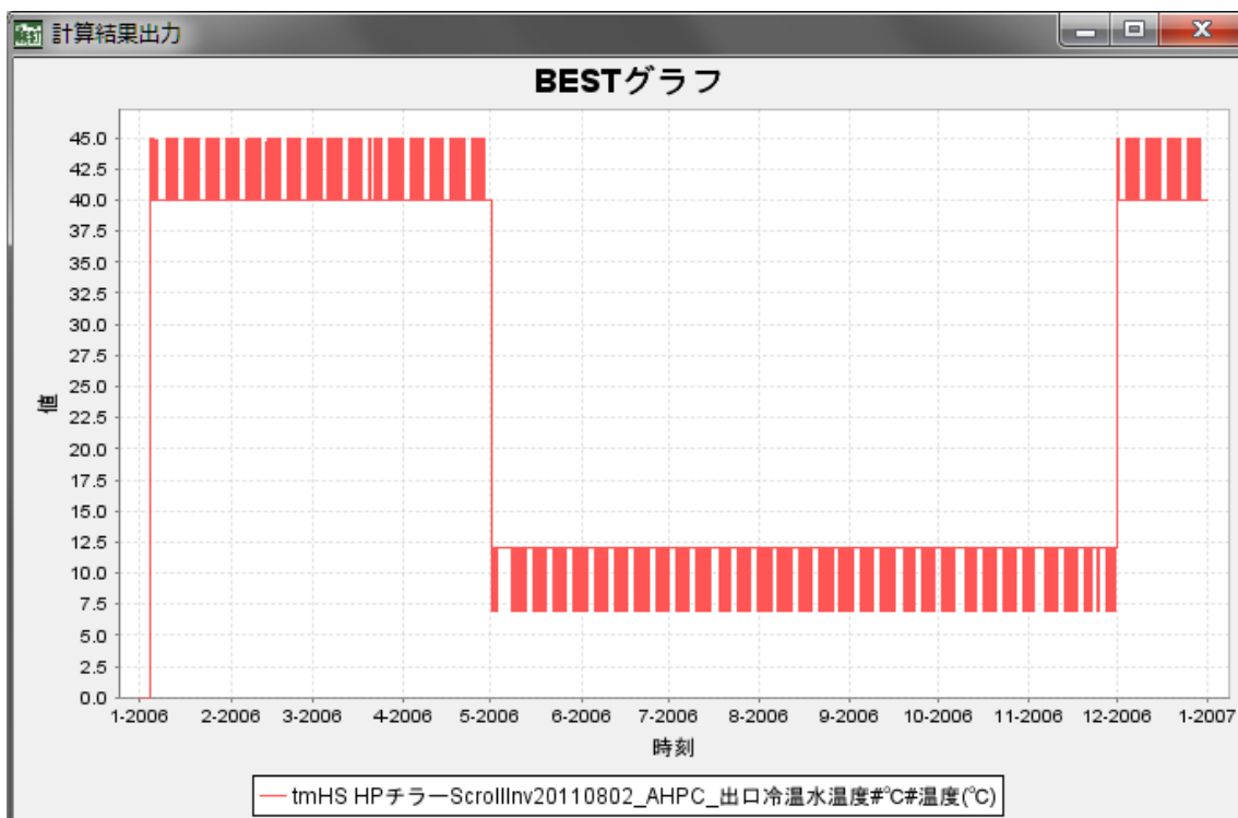
図 5-28 熱源 (HP チラー) のデフォルトでの計算結果 年間の熱源出口冷温水温度
