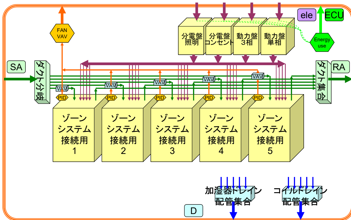
図 4-1 ゾーンテンプレートの実装例(ゾーンを5個含む例)
