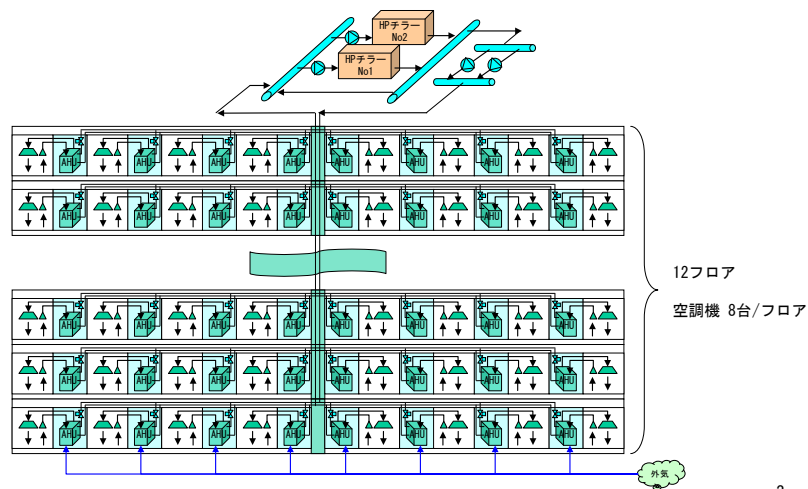
図 3-84 熱源と空調系統のモデルの概要
