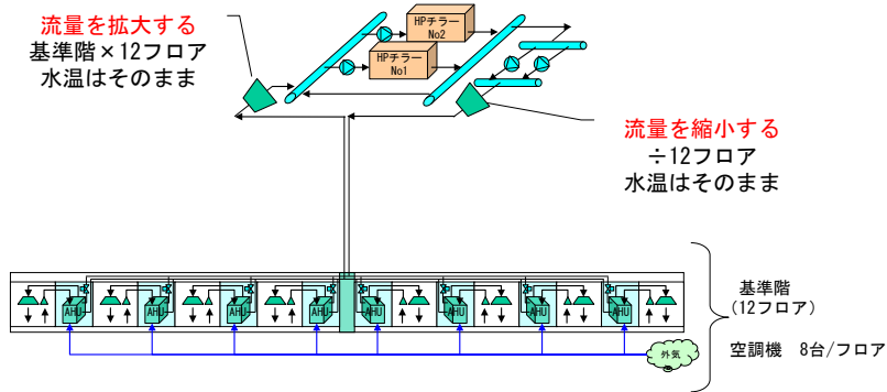
図 3-85 熱源と空調系統のモデルの概要 (基準階)
