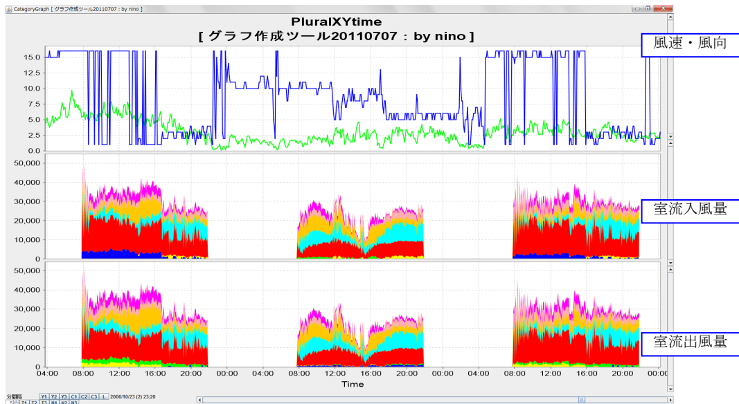
図 5-16 計算結果(3)
