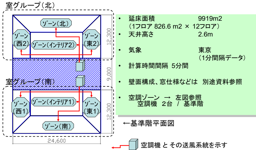
図 3-2 建築モデルの基準階ゾーンと2次側の空調設備
