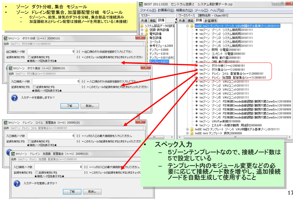
図 3-20 ゾーンテンプレートを構成モジュール(3)
