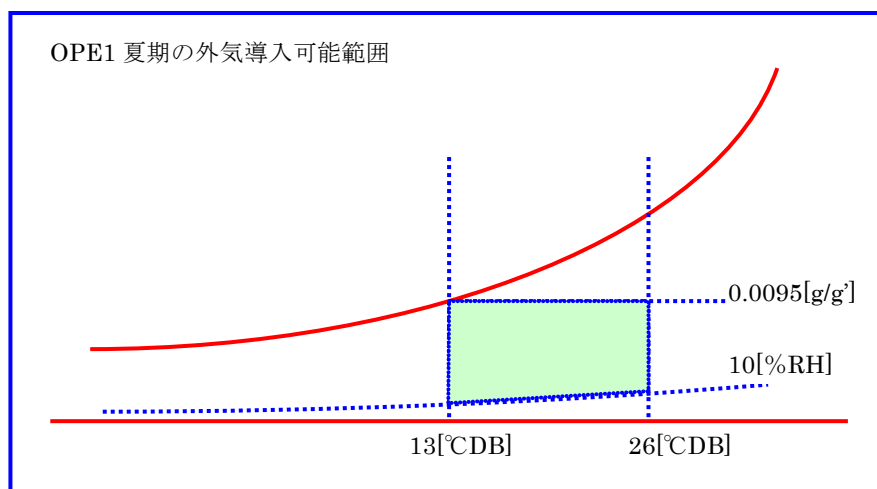
図 5-20 外気冷房時の外気導入条件/OPE1 夏期の例
