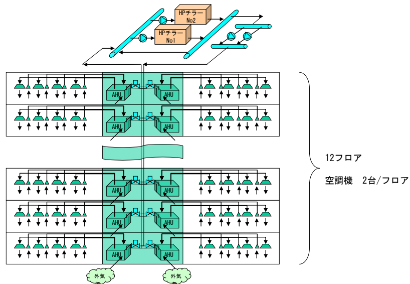
図 3-3 2次側空調設備と熱源
