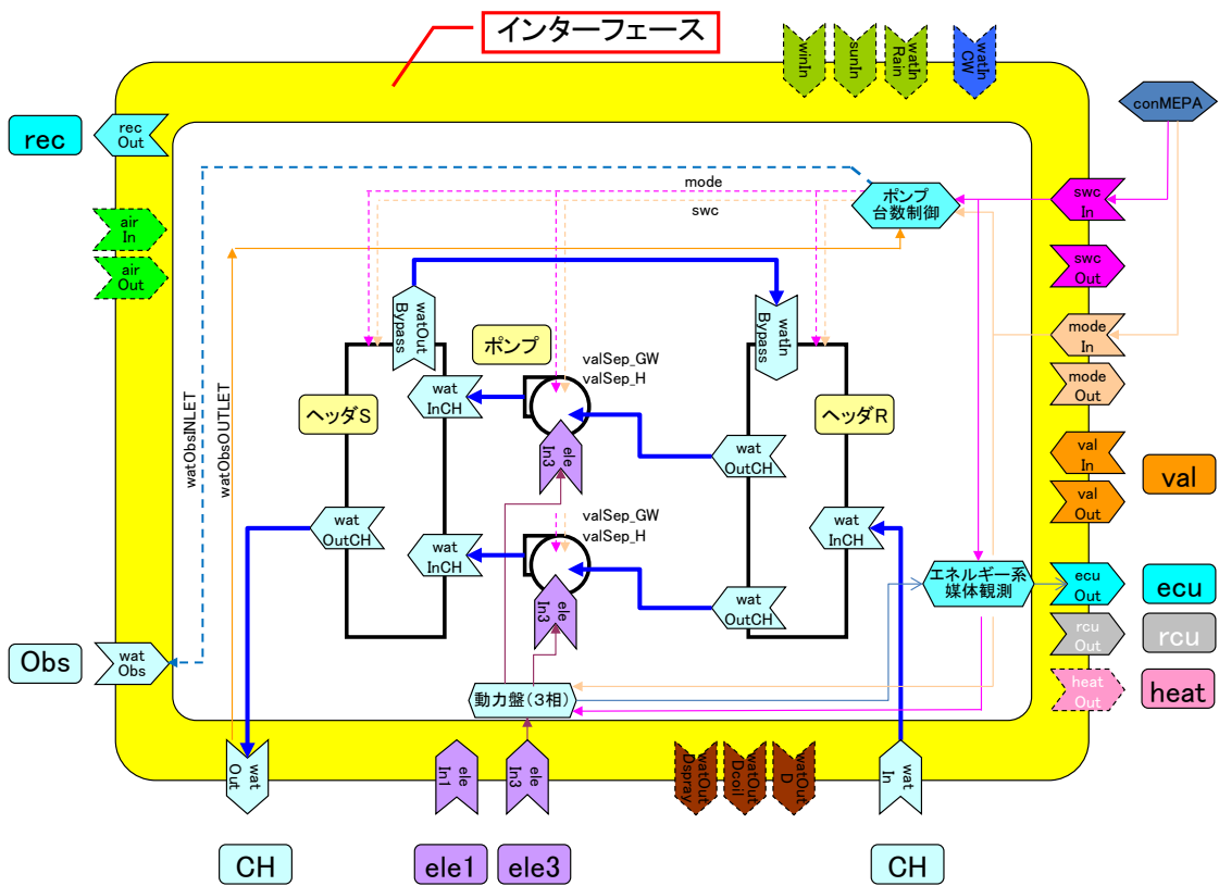
図 4-30. 「ゾーン空調プレート」の内部構成の参考詳細図
