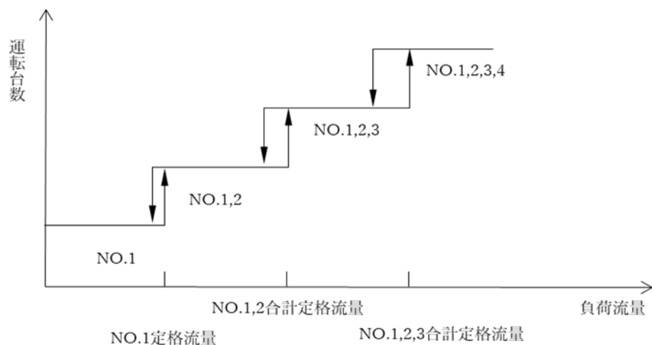
図 4-34. ポンプ台数制御の概要(4台の場合)
