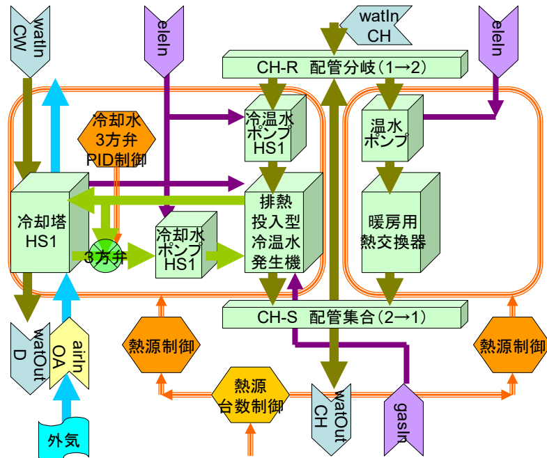
図 3-68 熱源廻りの構成部品 (モジュール)
