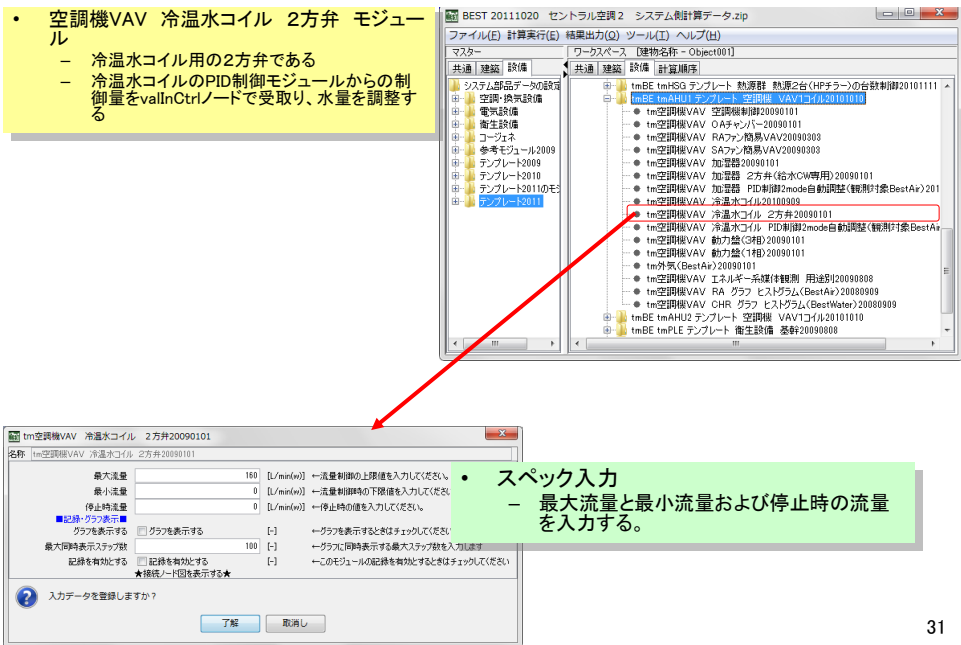
図 3-35 空調機テンプレート構成モジュール(8)
