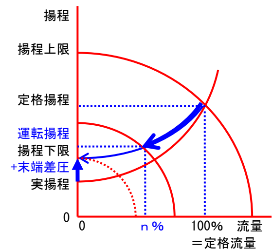
图 5-49 末端差压一定制御
