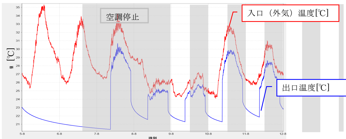
図 5-6 アースチューブの入口・出口温度の週変動(夏季:8/5~12)
