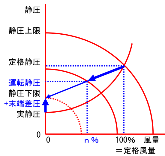
図 5-60 予想末端差圧制御
