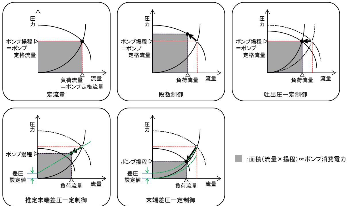
図 4-29. 2次ポンプの変流量制御による省エネ効果
