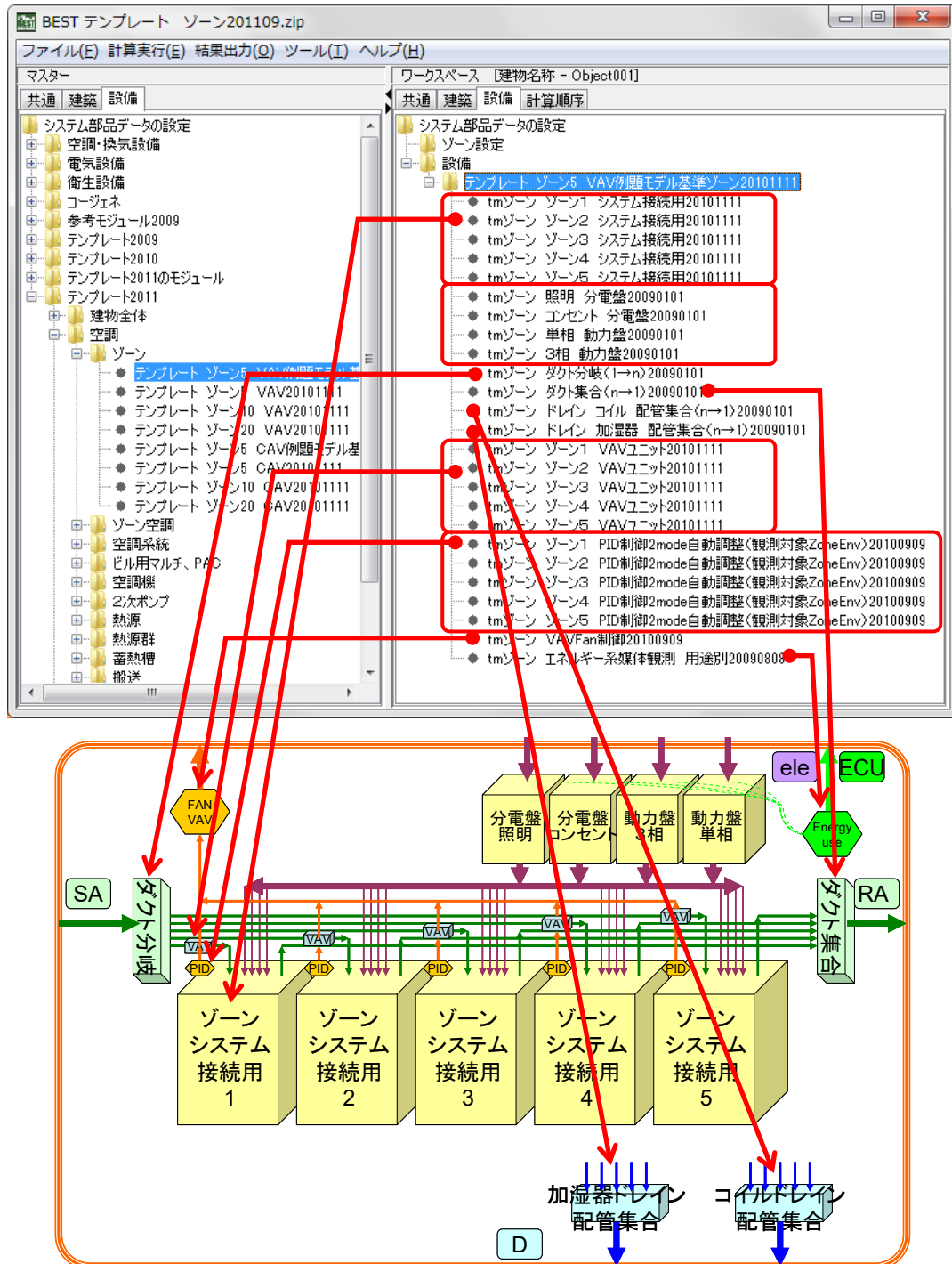
図 4-3 テンプレートを構成するモジュール
