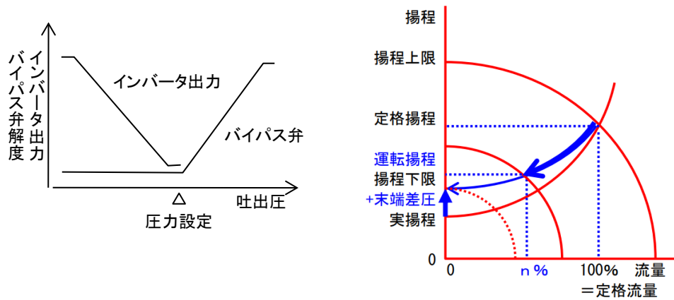
図 4-36. 末端差圧一定制御の概要
