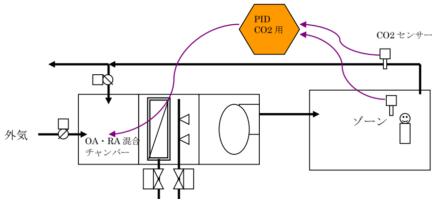
図 5-17 空調機 CO2 濃度制御の空調設備モジュールの構成の例
