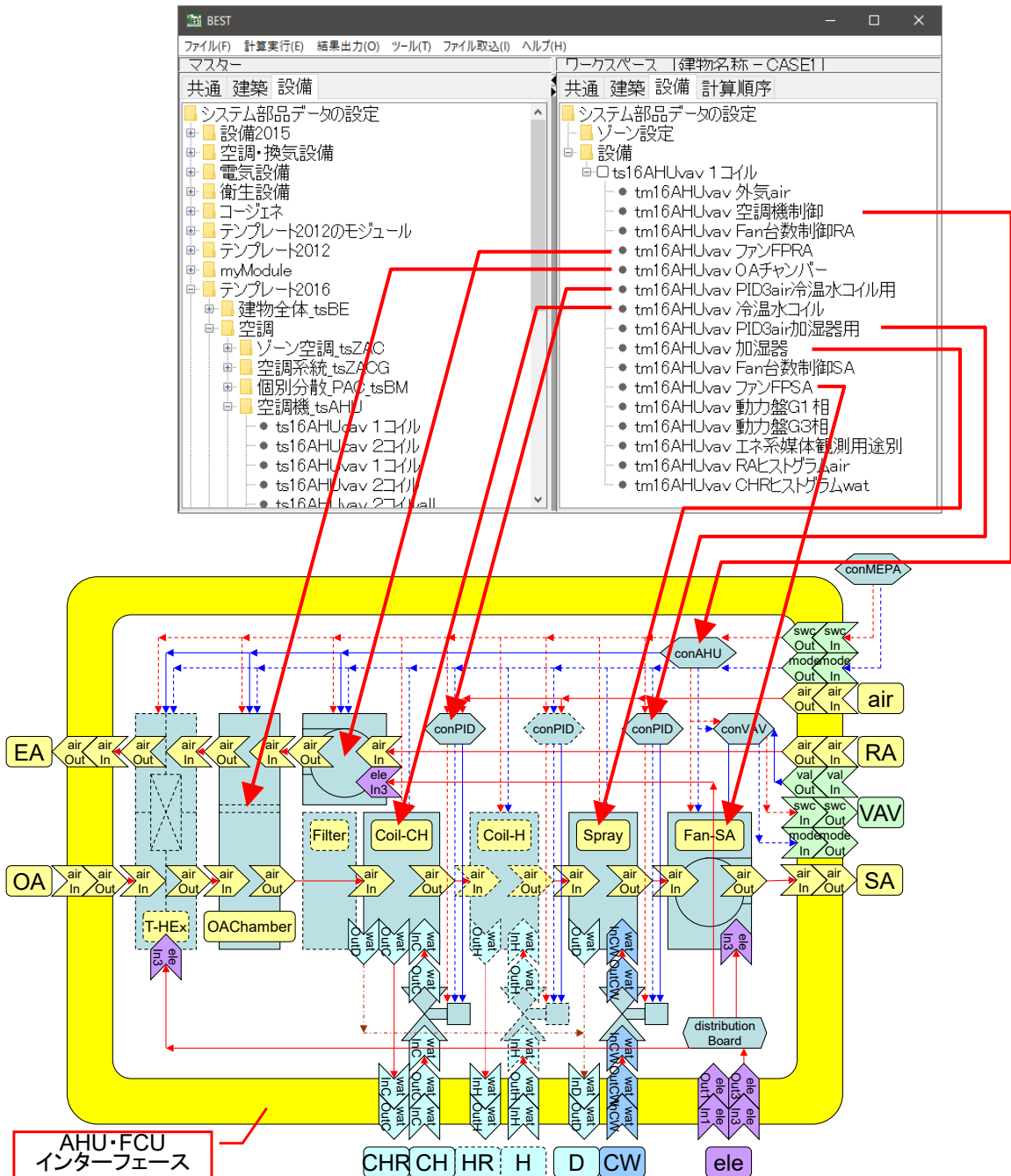
図 4-27 モジュール構成と内外接続と入出力の関係
