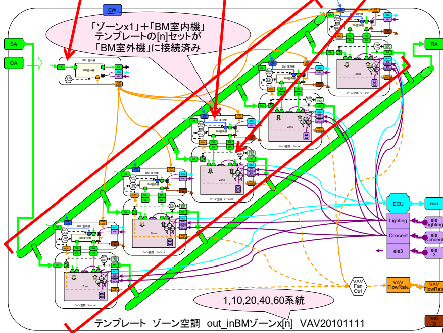
図 4-16 テンプレート ゾーン空調 out_inBM ゾーン x5 VAV20101111
