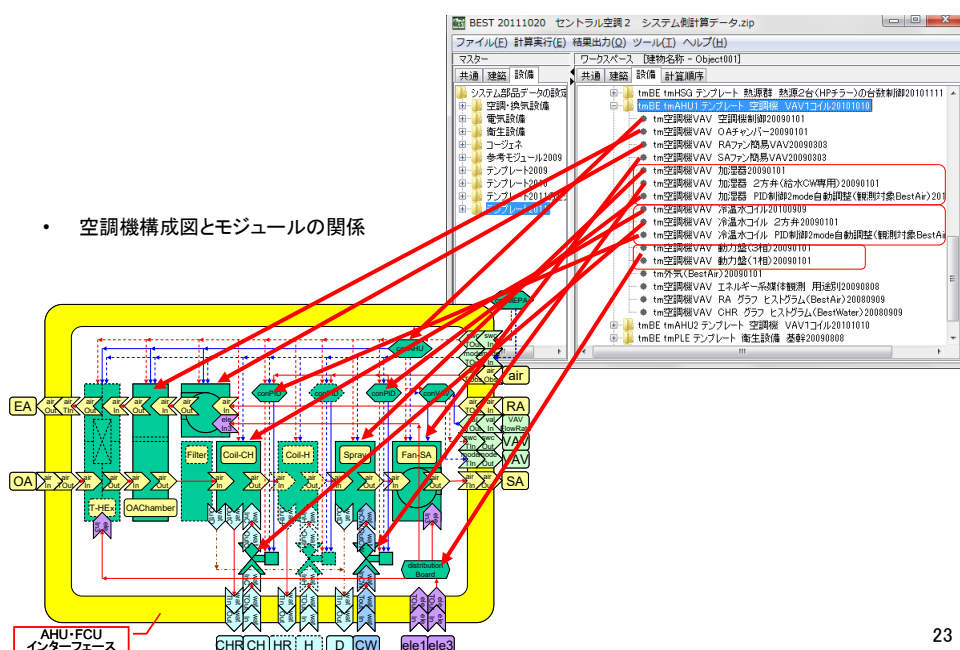
図 3-27 空調機テンプレートを構成するモジュール
