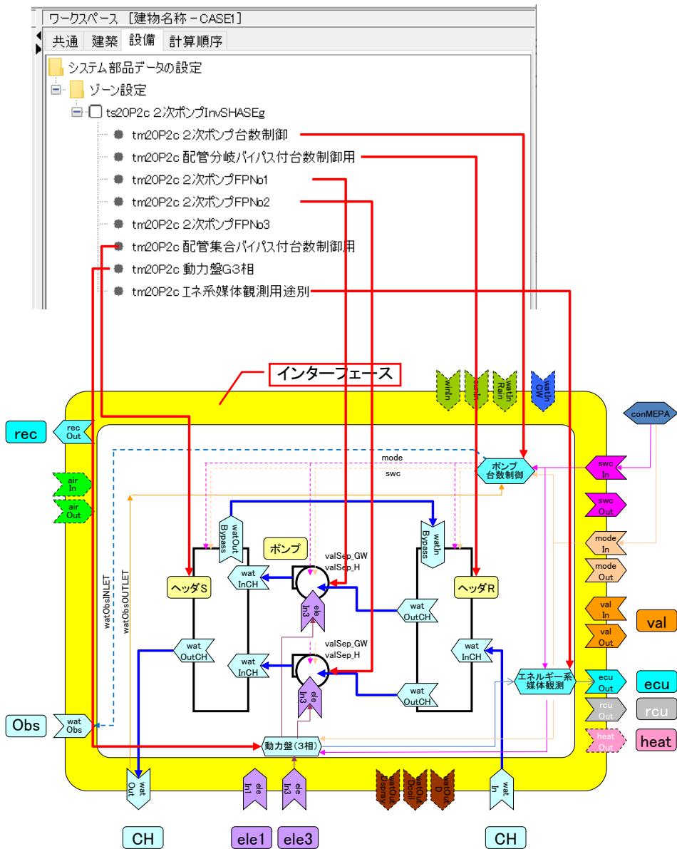
図 4-32. モジュール構成と内外接続と入出力の関係
