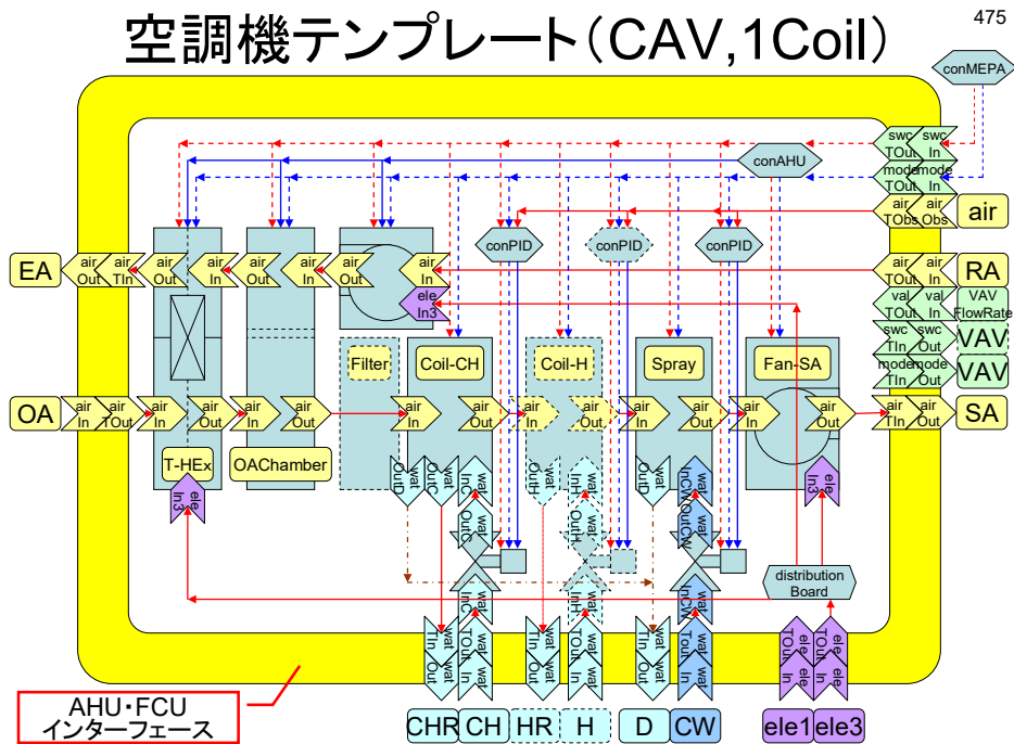
図 3-1 空調機テンプレート
