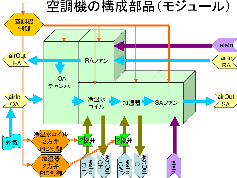
図 3-25 空調機の構成部品(モジュール)
