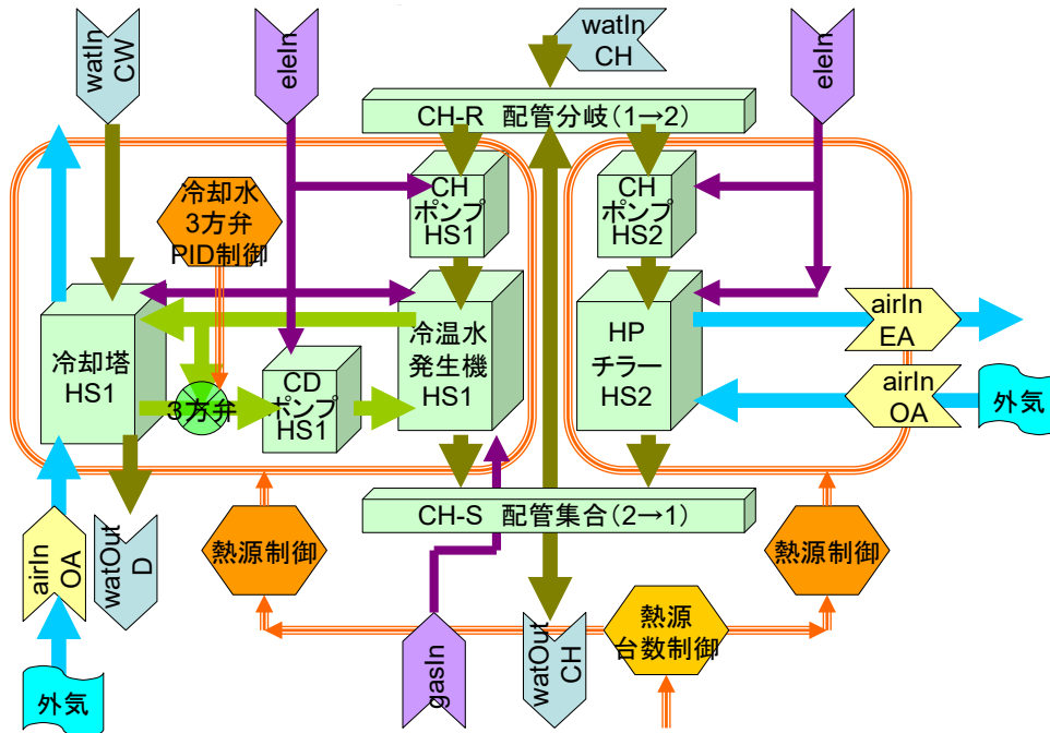
図 3-77 熱源廻りの構成部品(モジュール)
