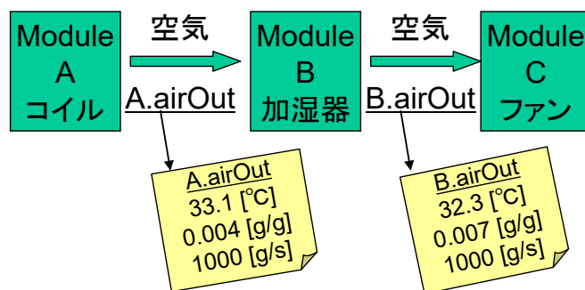
図 5-63 空気の状態値をオブジェクトで受渡す場合
