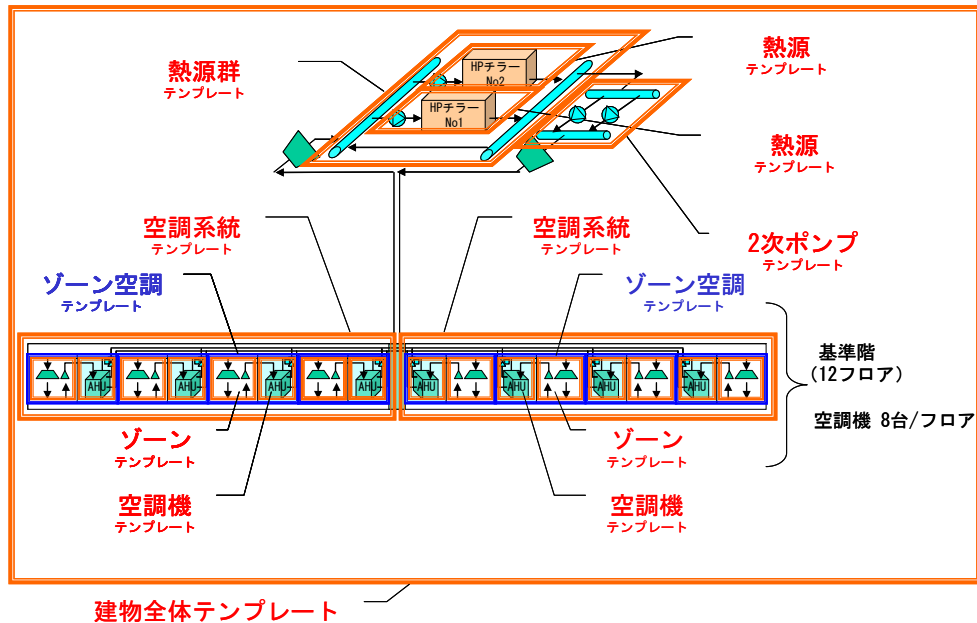
図 3-86 基準階のテンプレート構成
