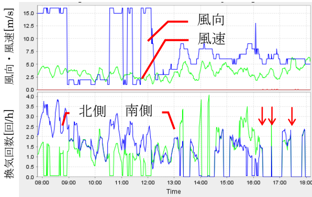
図 5-9 換気計算の結果(5/24 8:00~18:00)
