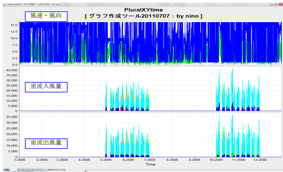
図 5-14 計算結果(1)
