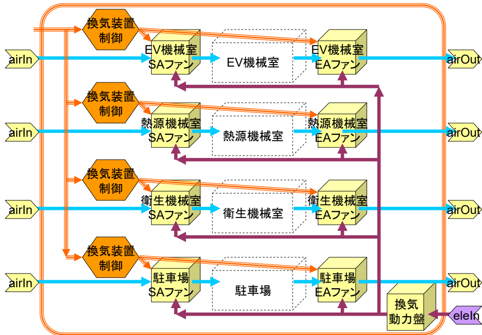
図 3-59 換気設備の構成部品(モジュール)
