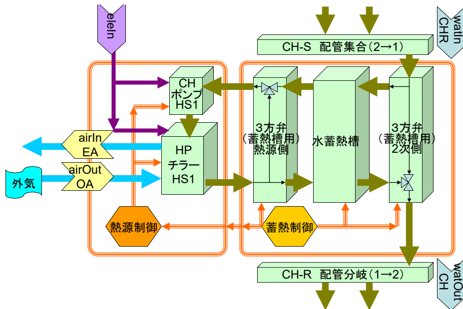
図 3-65 熱源廻りの構成部品 (モジュール)
