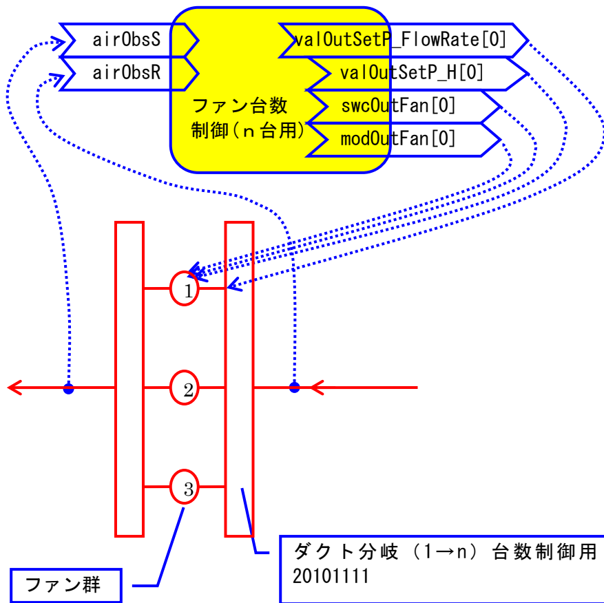
図 5-55 ノードの接続例 ポンプ群
