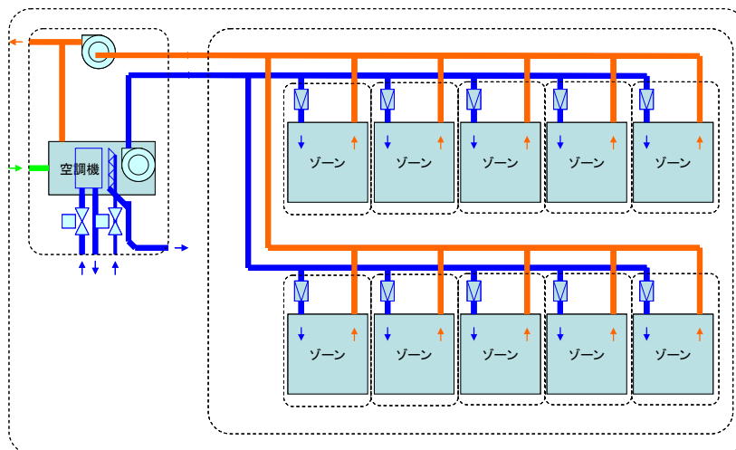
図 4-6 ゾーン空調テンプレートの特徴(実装例) (空調機の送風系統のゾーン数を簡単に変更できる)
