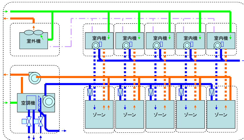
図 4-9 ゾーン空調プレートの特徴(実装例) (空調機+ビル用マルチの2次側複合システムの構築)
