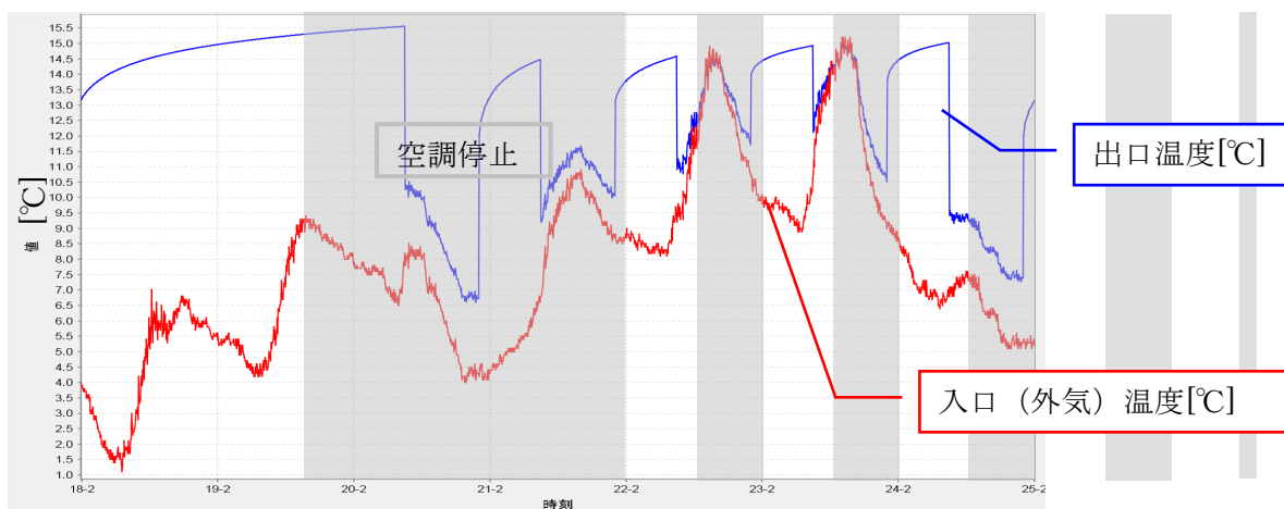
図 5-5 アースチューブの入口・出口温度の週変動(冬季:2/18～24)
