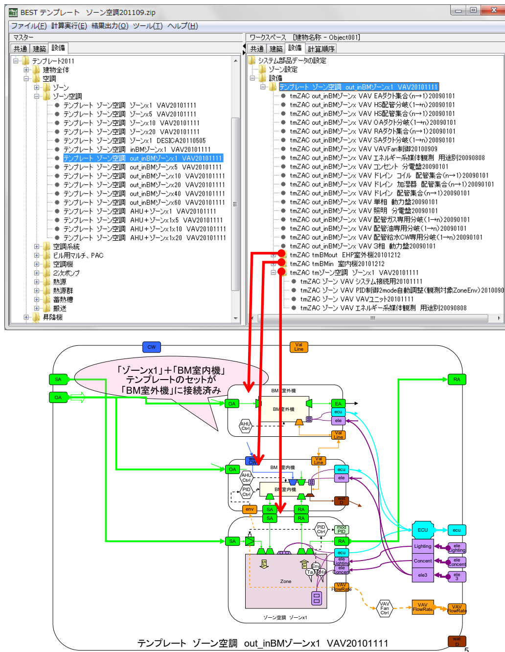
図 4-15 テンプレート ゾーン空調 out_inBM ゾーン x1 VAV20101111
