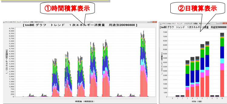
図 3-12 建物全体テンプレート直下の主なモジュール(4)
