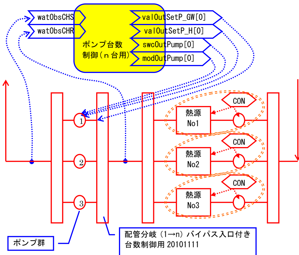
図 5-45 ノードの接続例 ポンプ群
