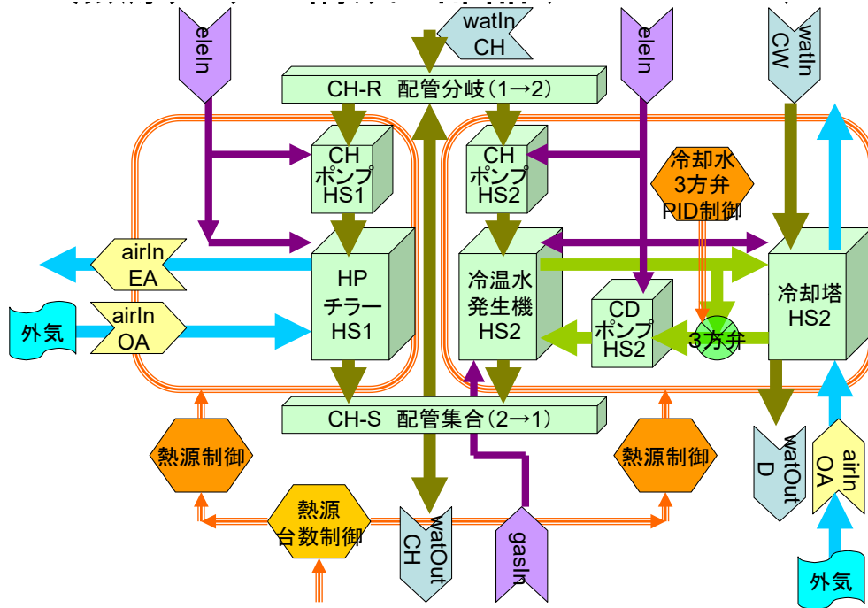
図 3-75 熱源廻りの構成部品(モジュール)
