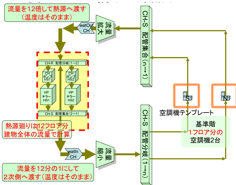
図 3-42 2次側ヘッドと熱源廻りの構成
