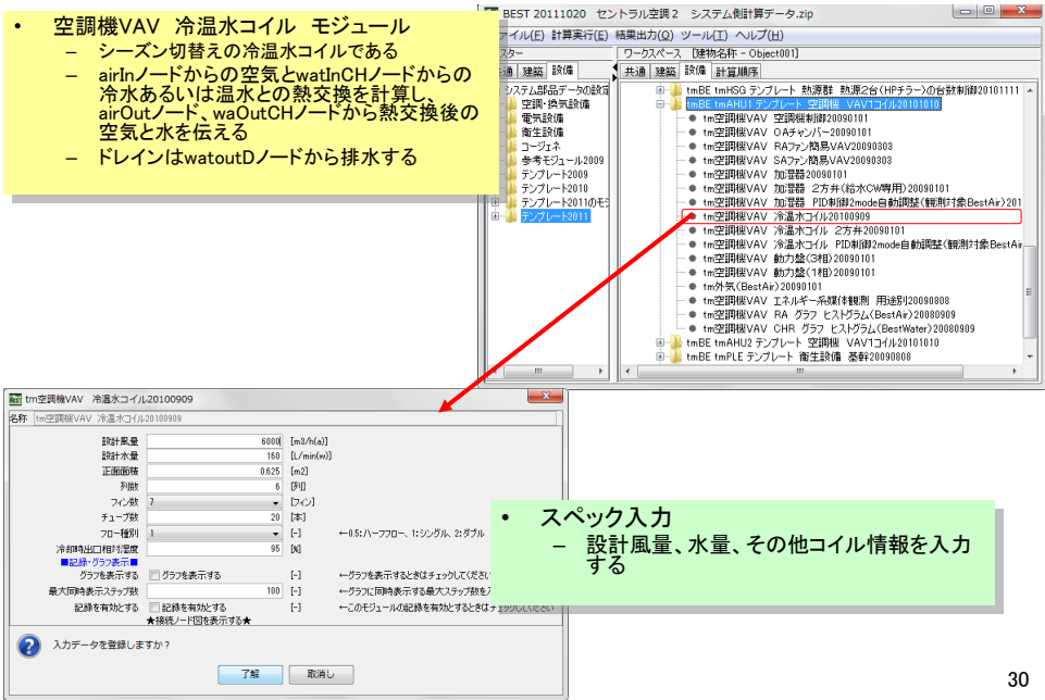
図 3-34 空調機テンプレート構成モジュール(7)
