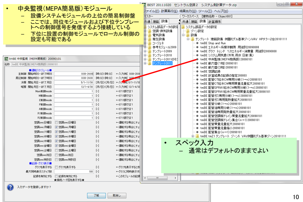
図 3-10 建物全体テンプレート直下の主なモジュール(2)
