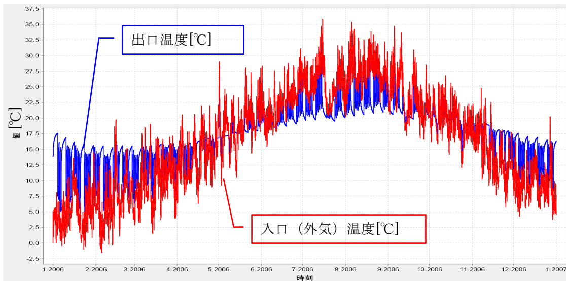
図 5-4 アースチューブの入口・出口温度の年変動
