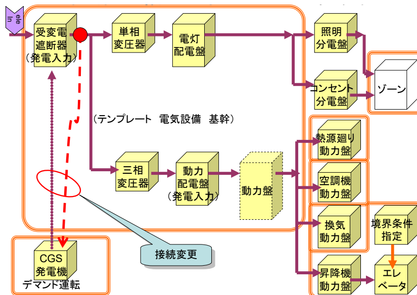
図 3-72 電気設備の構成部品(基幹 変更後)
