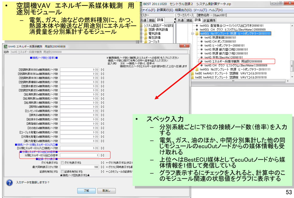
図 3-56 熱源テンプレート構成モジュール(6)
