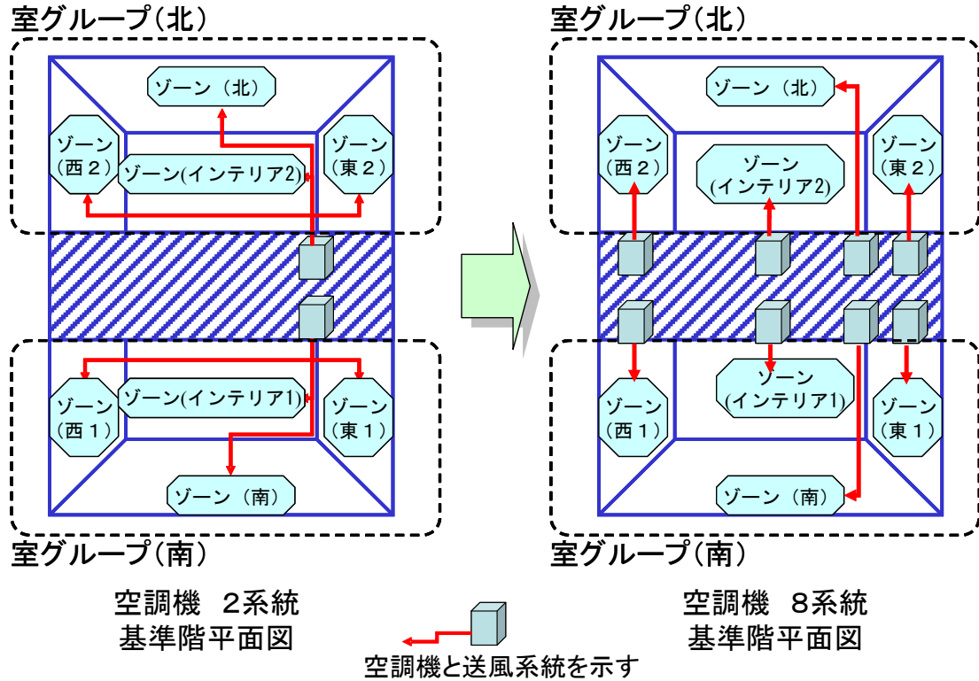
図 3-83 空調系統の変更内容
