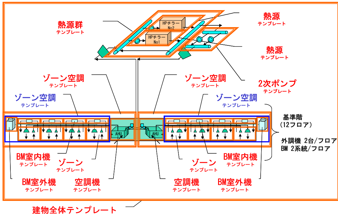
図 3-90 空調システムのテンプレート構成
