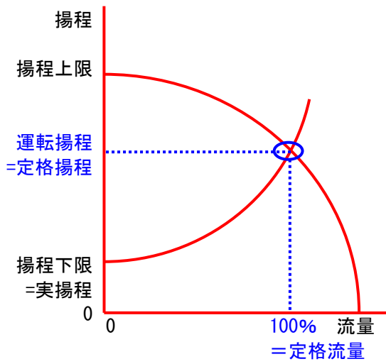
图 5-46 定流量
