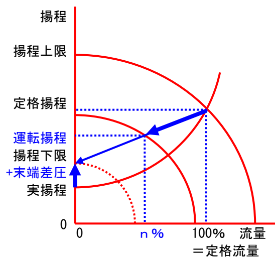
図 5-50 予想末端差圧制御
