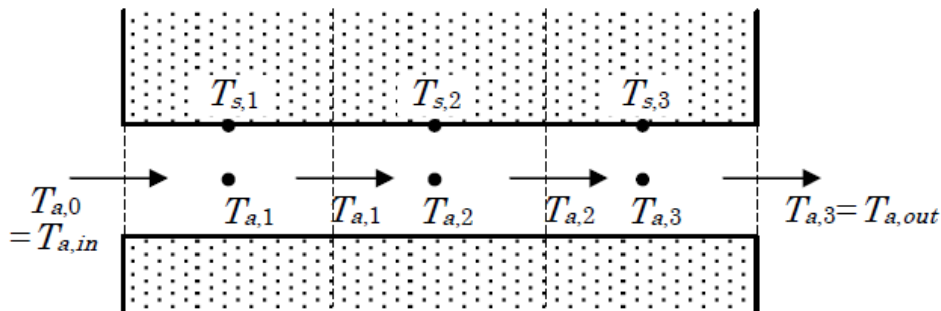
図 5-8 アースチューブの概要
