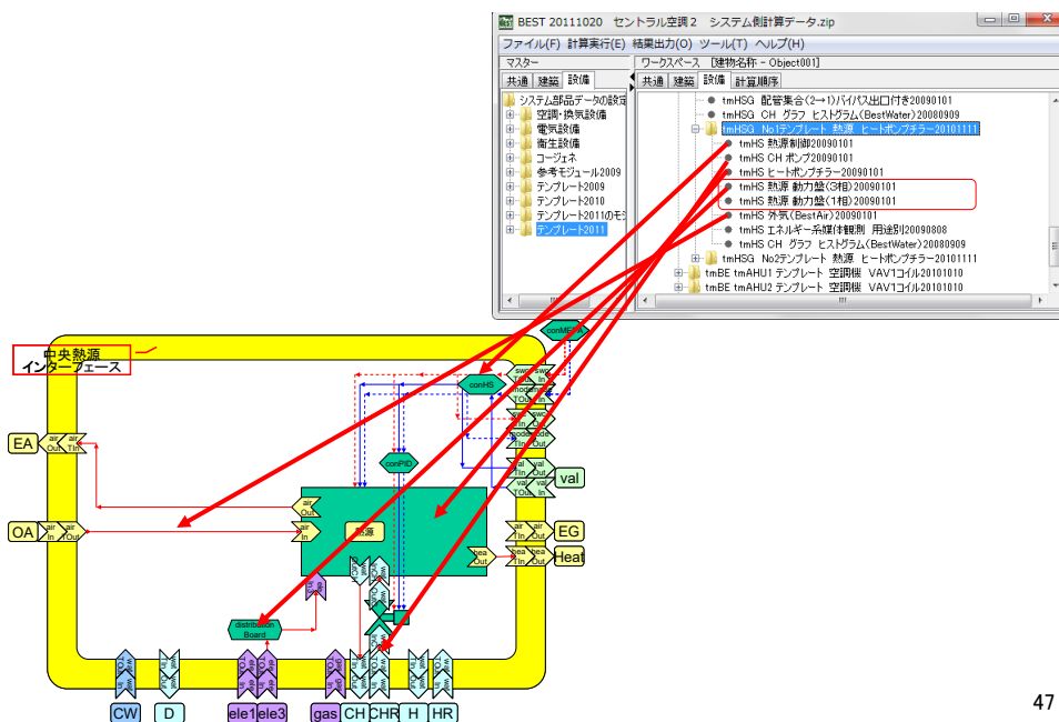
図 3-50 熱源テンプレート構成モジュール例
