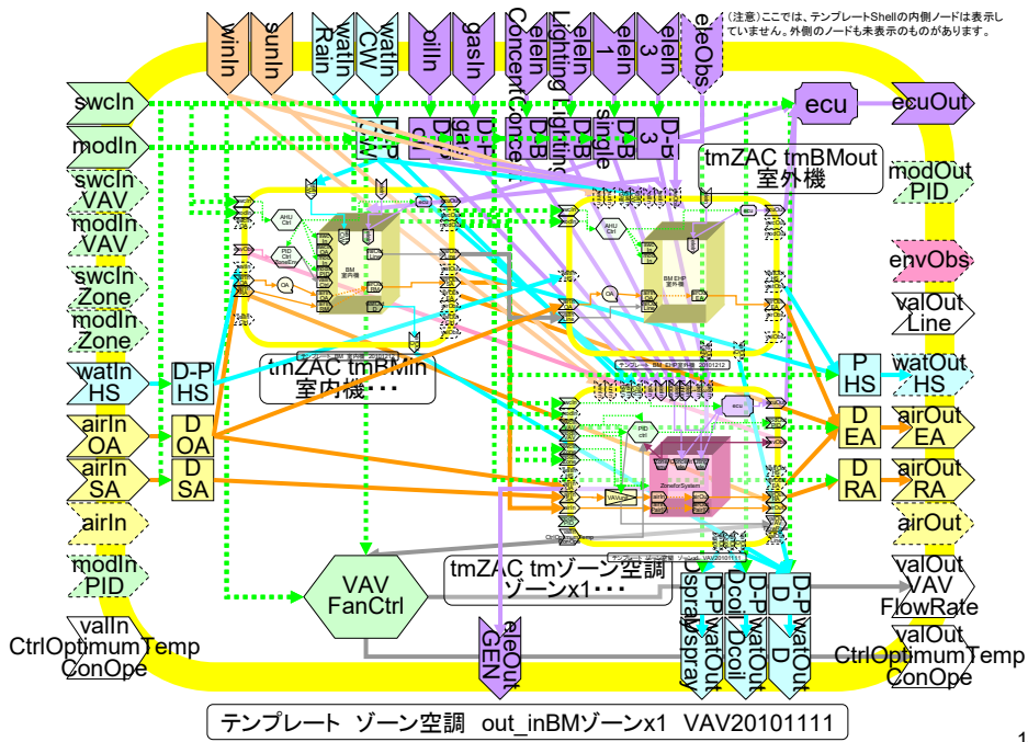
図 4-20「ゾーン空調テンプレート」の内部構成の参考詳細図(2)
