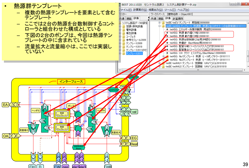
図 3-43 熱源群テンプレートを構成するモジュール
