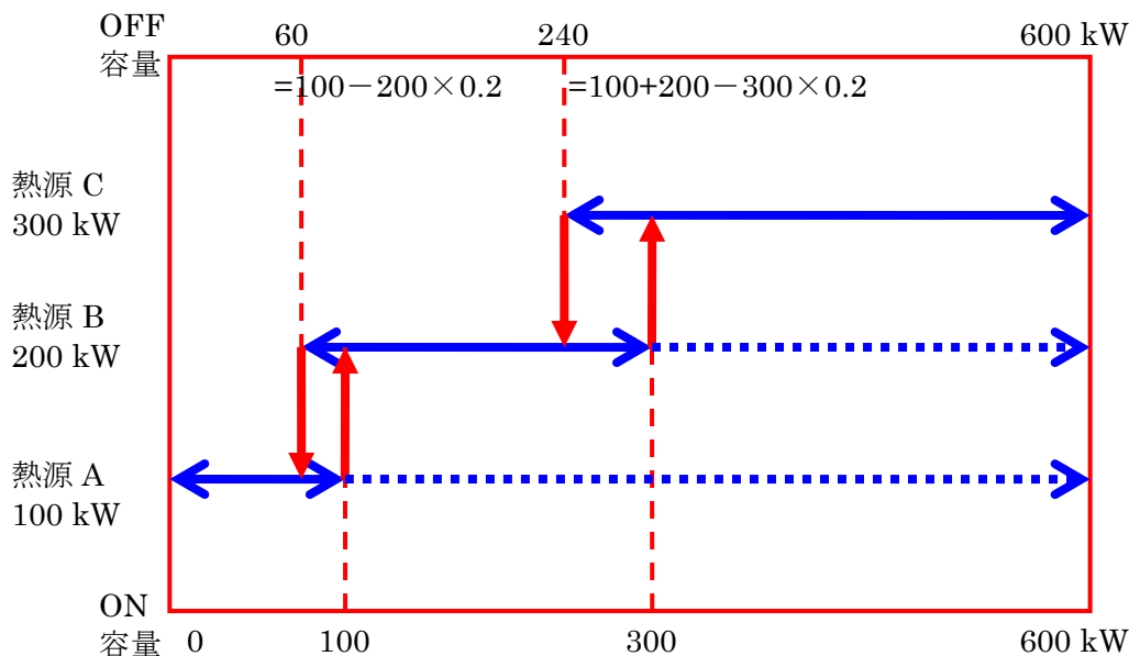
図 5-37 台数制御の例 [熱量による制御 定格容量 A=100、B=200、C=300kW]
