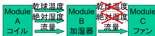
図 5-61 空気の状態値を個別に受渡す場合
