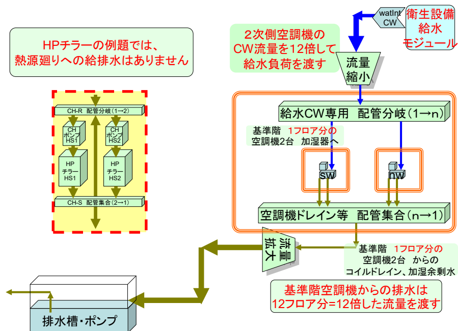
図 3-61 空調給排水の構成部品(モジュール)
