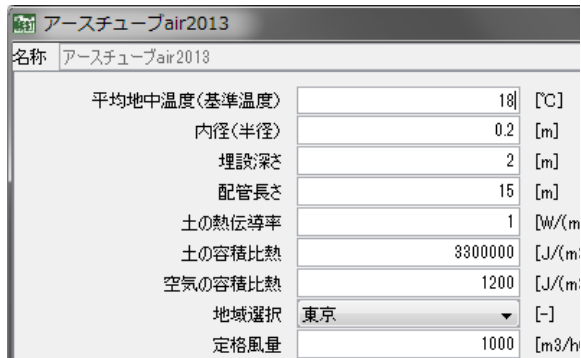
図 5-3 アースチューブの条件
