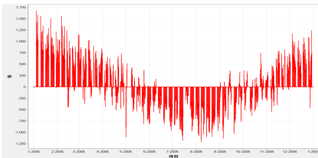
図 5-7 アースチューブの交換熱量の年変動
