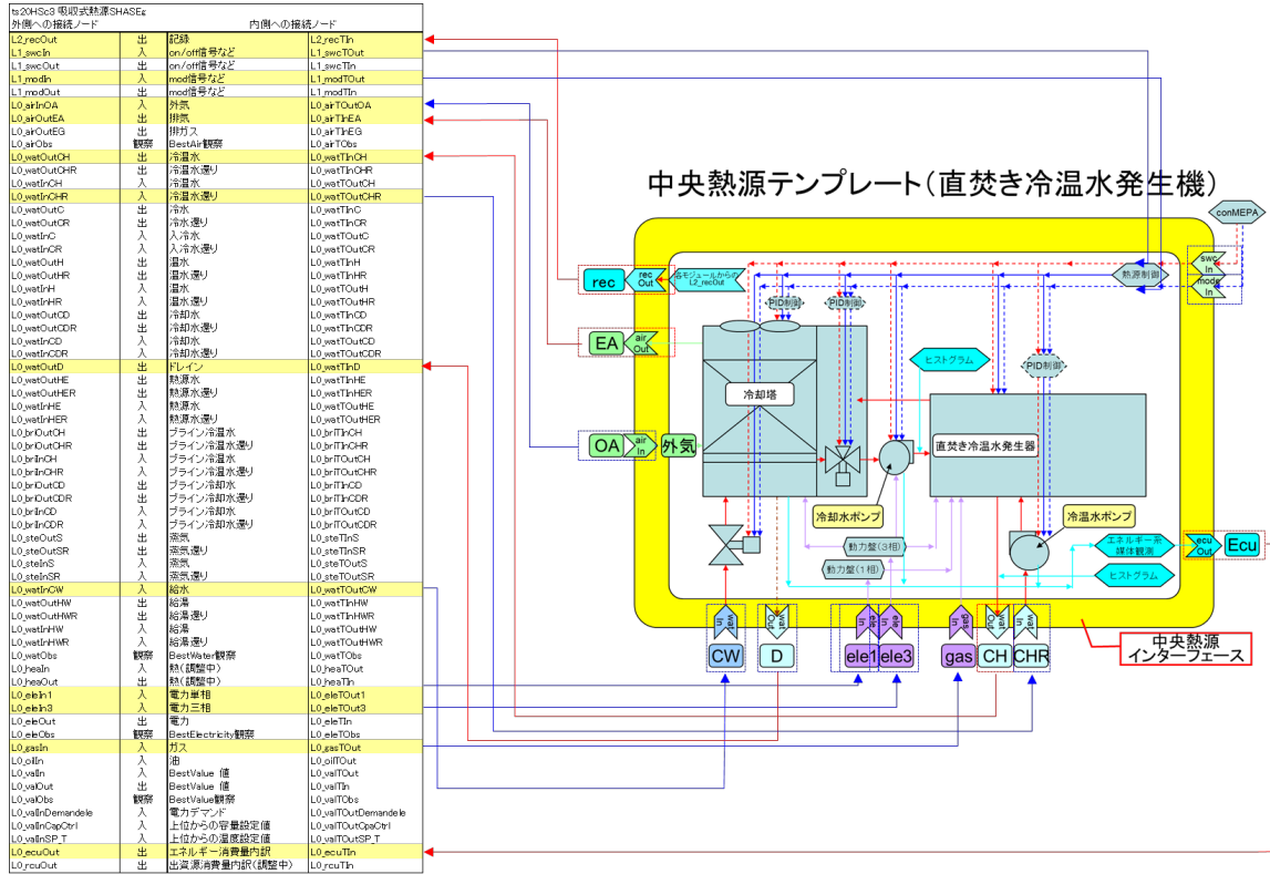
図 4-45 テンプレート「熱源」の Shell と内部モジュールとのノード接続情報 (テンプレート 熱源 ts20HSc3 吸収式熱源 SHASEg の例)
