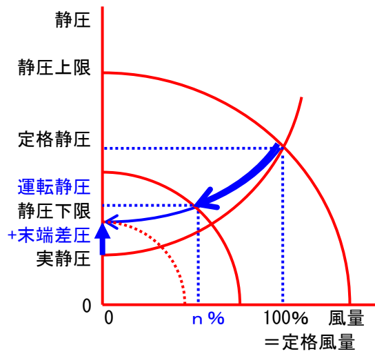
图 5-59 末端差压一定制御
