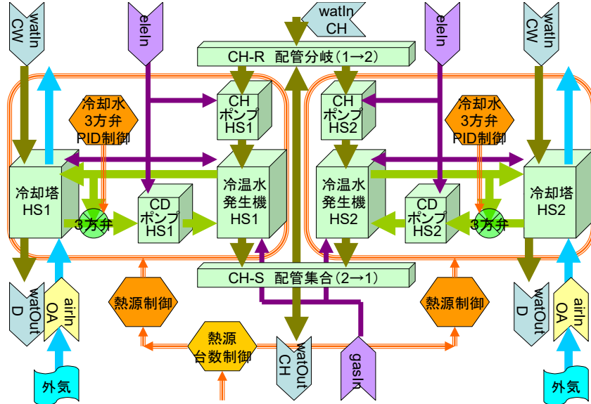
図 3-73 熱源廻りの構成部品(モジュール)
