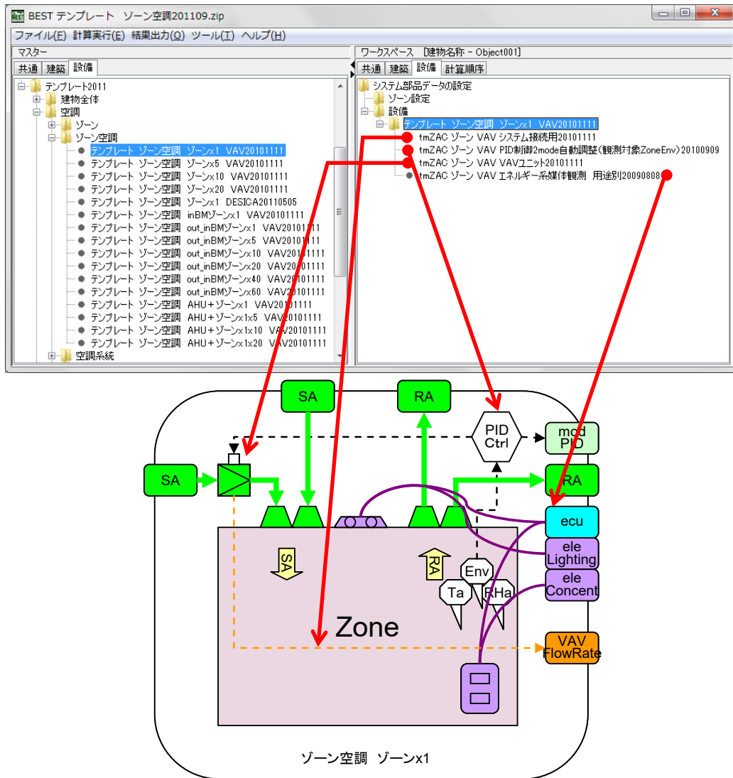
図 4-12 テンプレート ゾーン空調 ゾーン x1 VAV20101111
