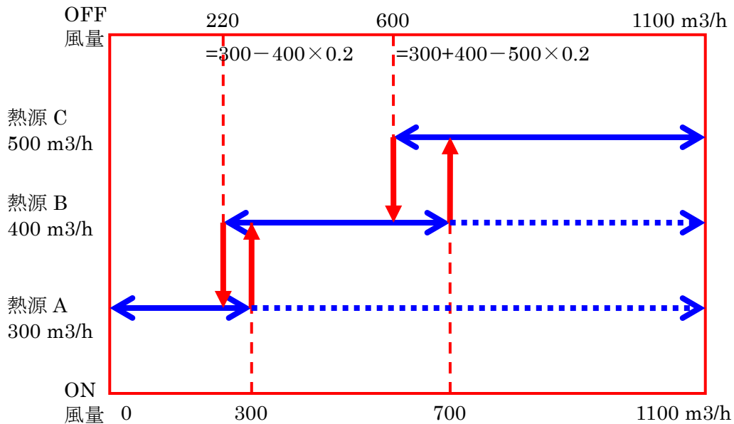
図 5-52 台数制御の例 [流量による制御 定格風量 A=300、B=400、C=500L/min]
