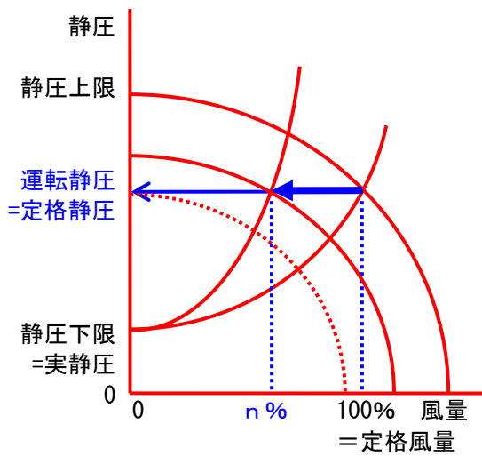
图 5-58 吐出压一定制御
