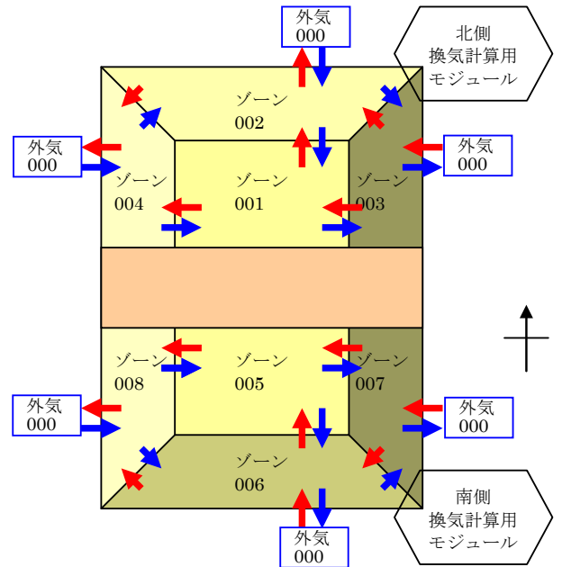
図 5-10 ゾーンと開口
