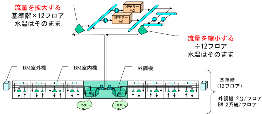
図 3-89 空調システムのモデル(基準階)
