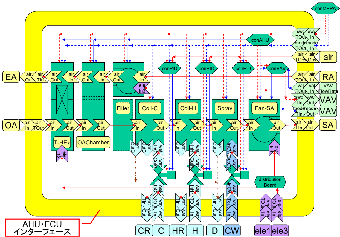
図 4-25「空調機テンプレート」の内部構成の参考詳細図
