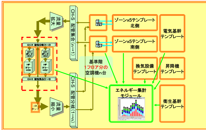
図 3-6 建物全体テンプレートの中の2次側空調設備テンプレートと熱源テンプレートの位置づけ
