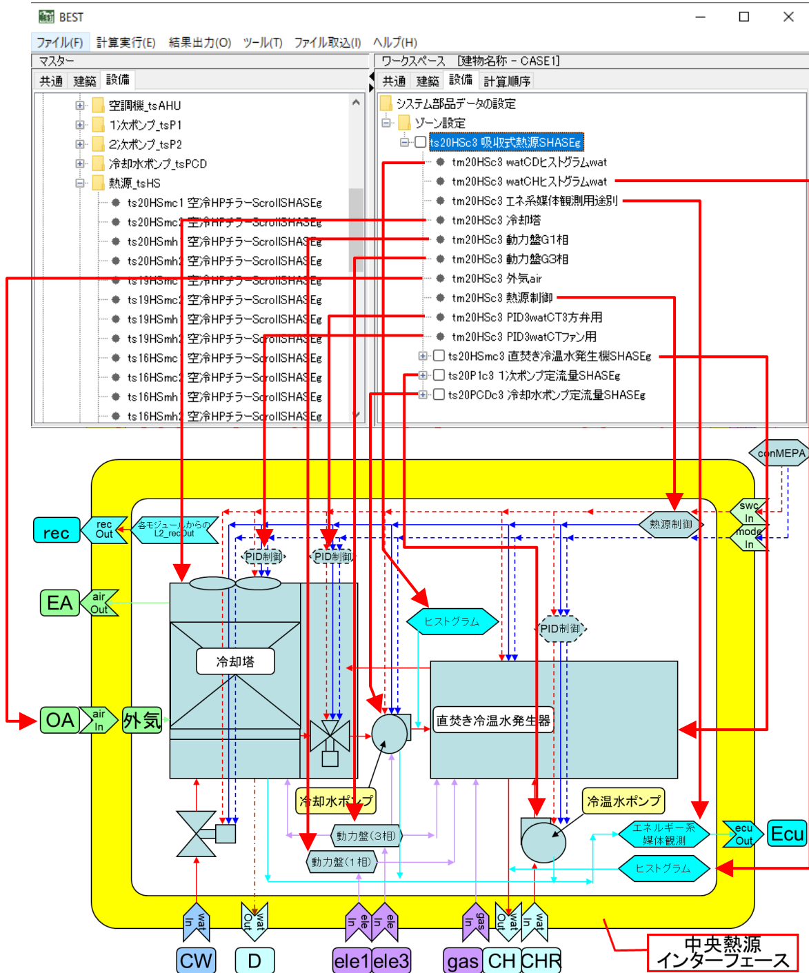
図 4-44 モジュール構成と内外接続と入出力の関係
