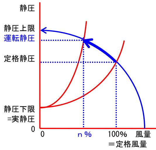
图 5-57 段数制御
