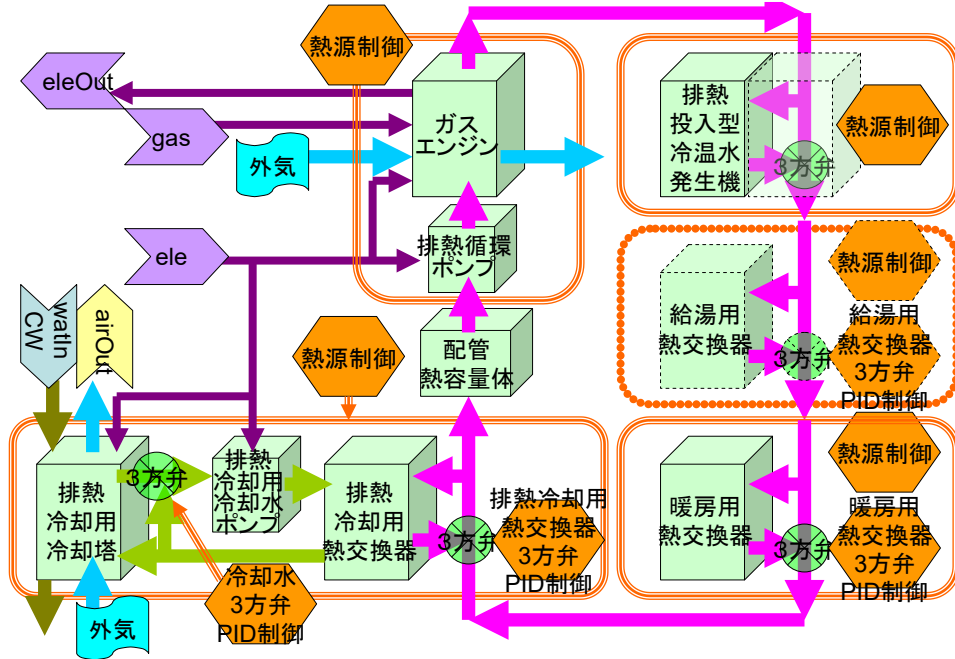
図 3-67 熱源廻りの構成 (排熱側部品) (モジュール)
