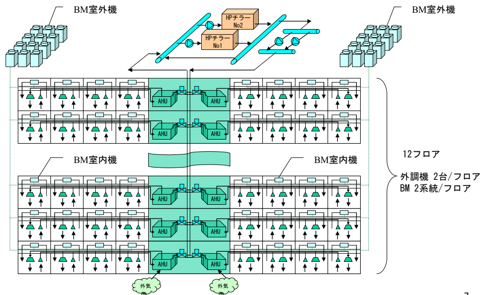
図 3-88 熱源と空調系統のモデルの概要
