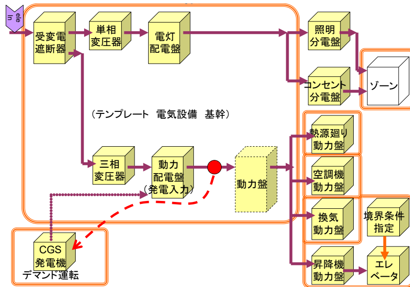
図 3-71 電気設備の構成部品(基幹)
