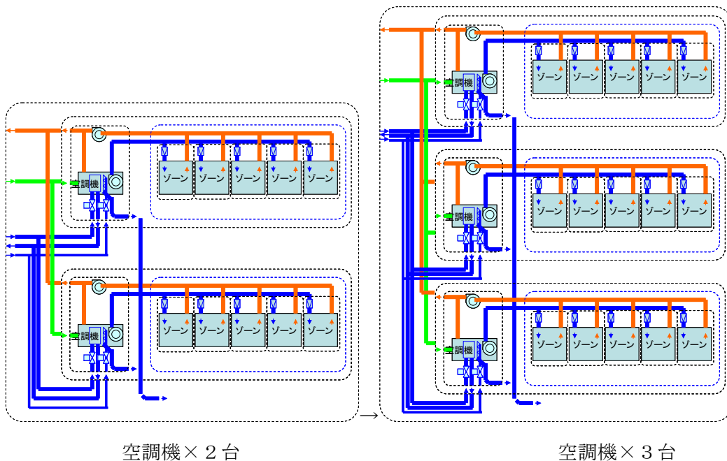
図 4-23「空調系統テンプレート」の実装例
